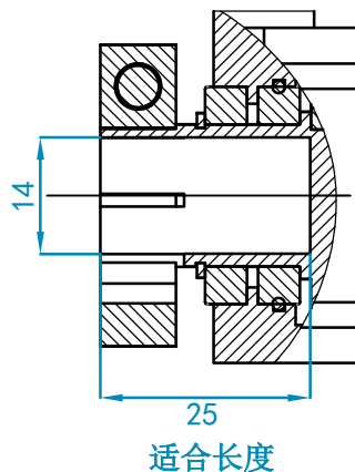
减速机输出轴剖面图
