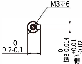
轴端规格
