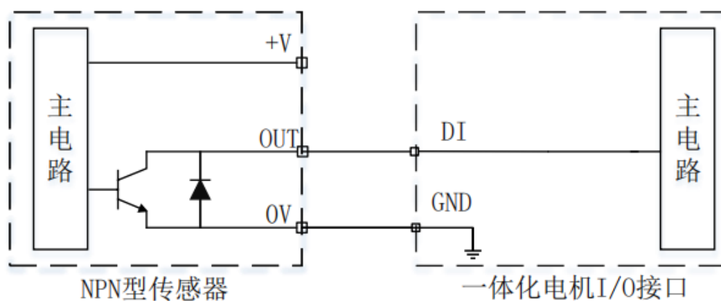
图 2-5 DI 输入端口接传感器输入（NPN）示意图
