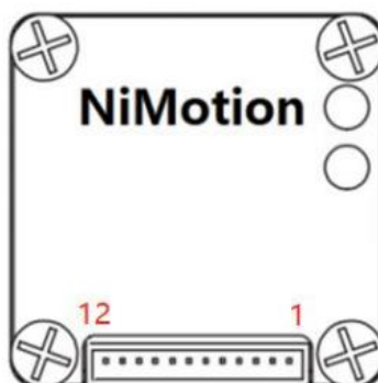
图 2-3 数字量输入输出 (I/O)、通信端口
