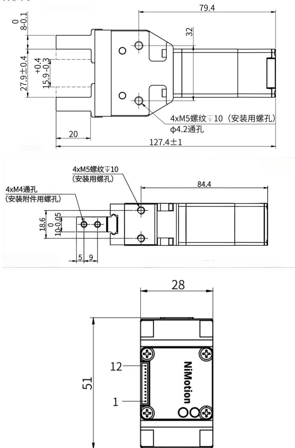
图 1-2 电动夹爪产品整机结构图
