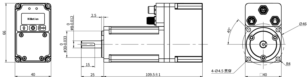
图 1-2 产品结构图
