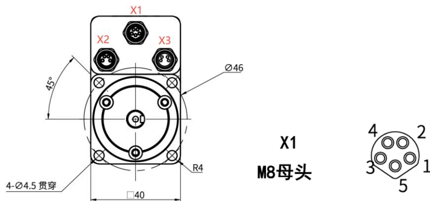
图 2-1 电源端口
