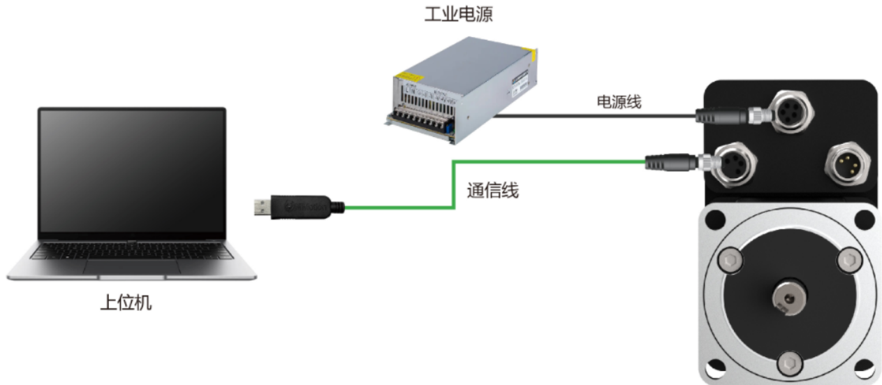
图 3-3 执行器调试（RS485/CANopen 通信）接线图
