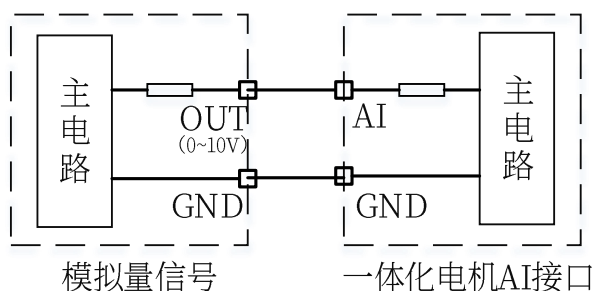
图 3-15 AI 端口接模拟量输入示意图
