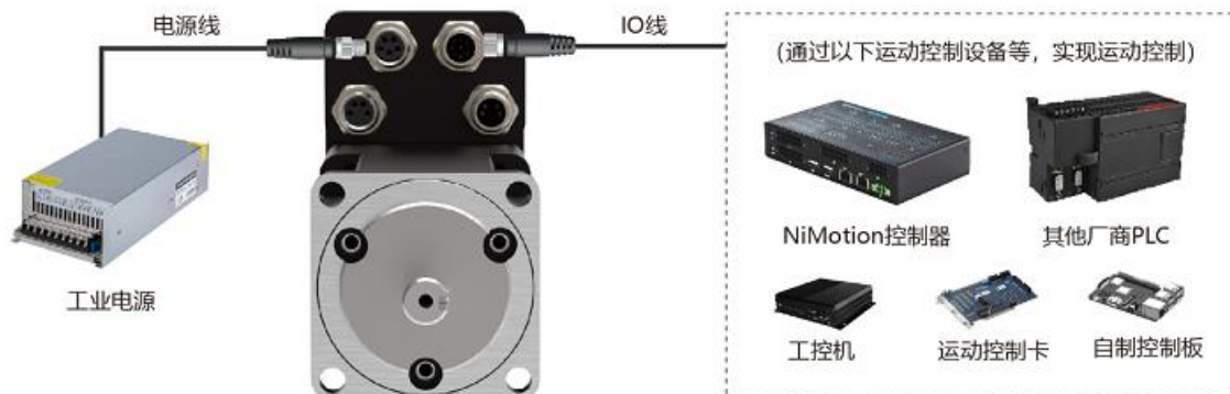
图 4-6 外部控制接线图（控制器通过 IO 端口控制）
