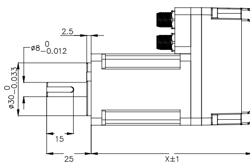
图 2-2 PMMP40 系列一体化电机结构图
