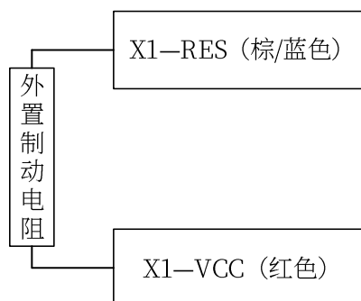
图 3-5 制动电阻接线图
