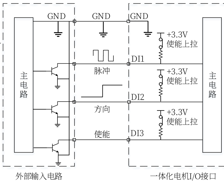
图 3-21 DI 输入端接脉冲示意图
