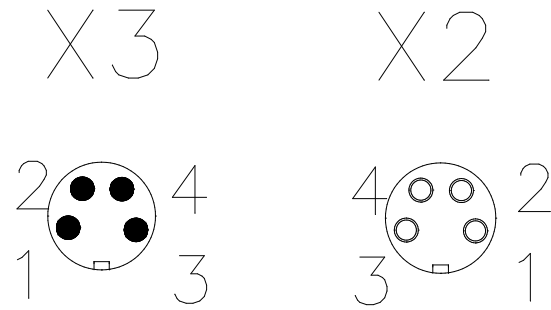
图 3-6 PMMP 系列通信线端口
