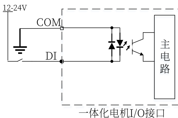
图 3-12 DI 输入端接开关示意图（共阴极）
