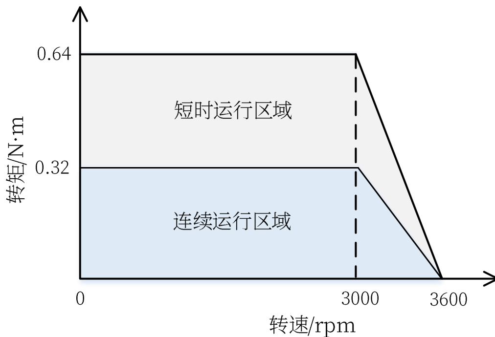
图 2-5 PMMP4010X-COE/CANopen/485-D03-X 矩频特性图 (48V, 3.20A)
