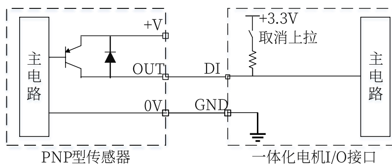
图 3-17 DI 输入端接 PNP 型传感器示意图
