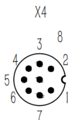
图 3-7 PMMP40 系列 I/O 端口
