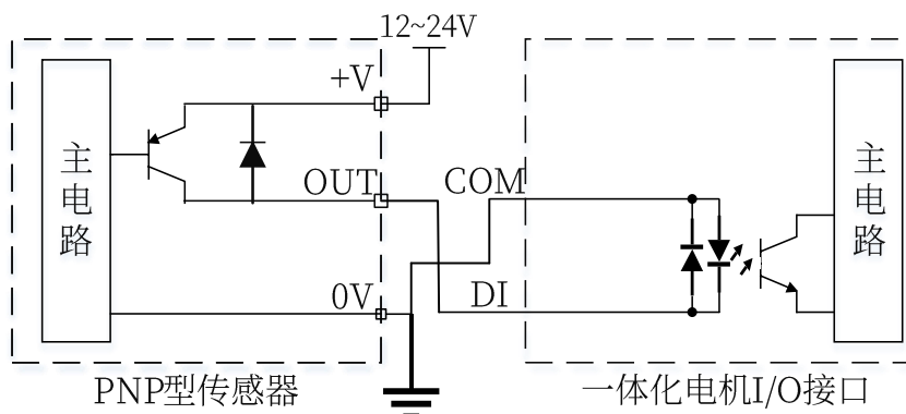
图 3-10 DI 输入端接 PNP 型传感器示意图
