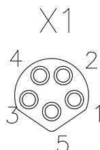
图 3-2 PMMP40 系列电源线端口
