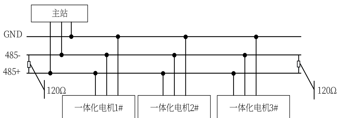
图 4-3 RS485 通信接线示意图
