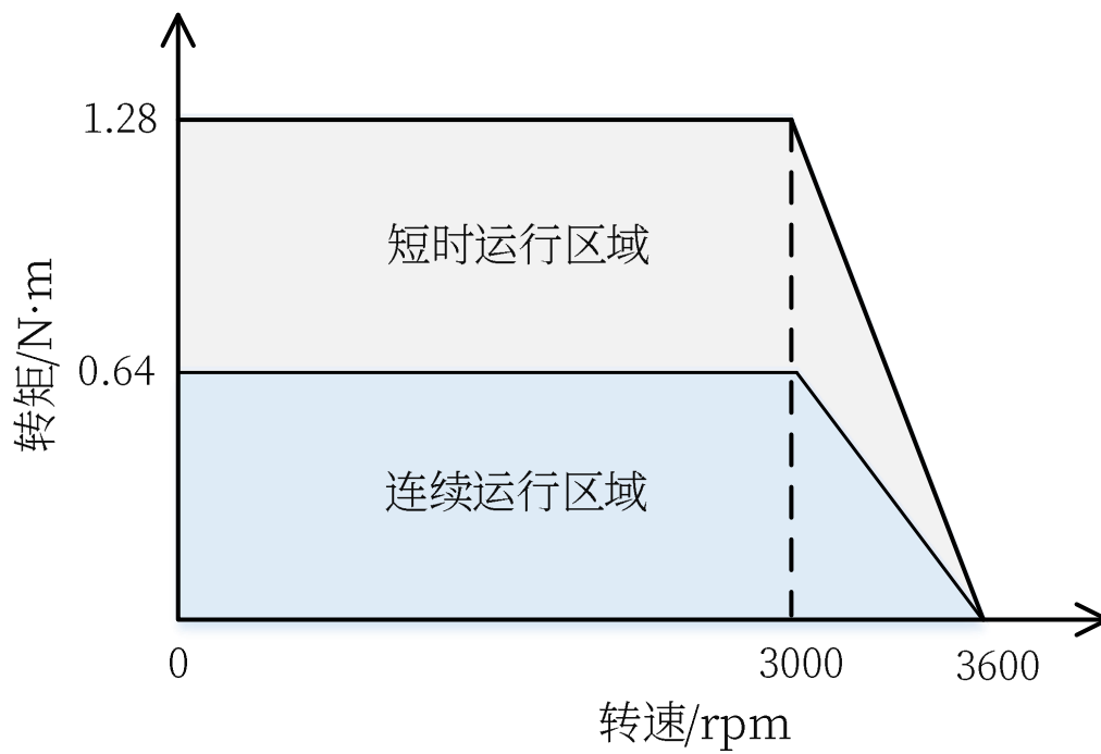
图 2-7 PMMP6020X-COE/CANopen/485-X 矩频特性图 (48V, 8.50A)
