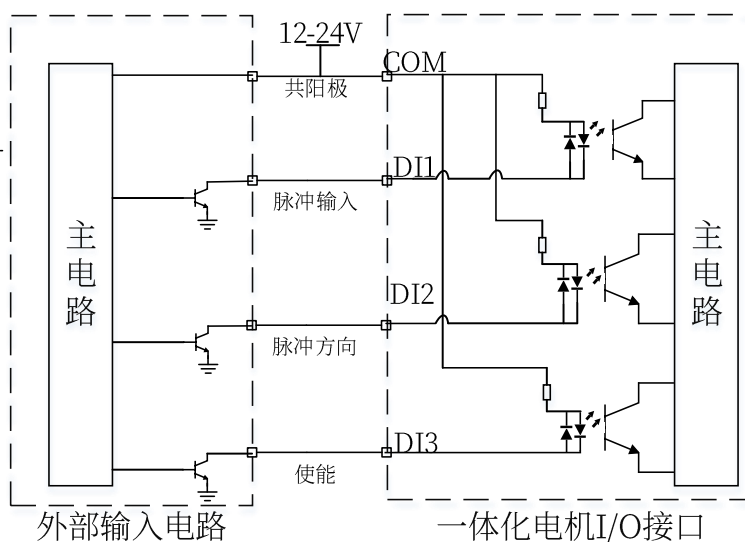
图 3-13 DI 输入端口接脉冲输入示意图
