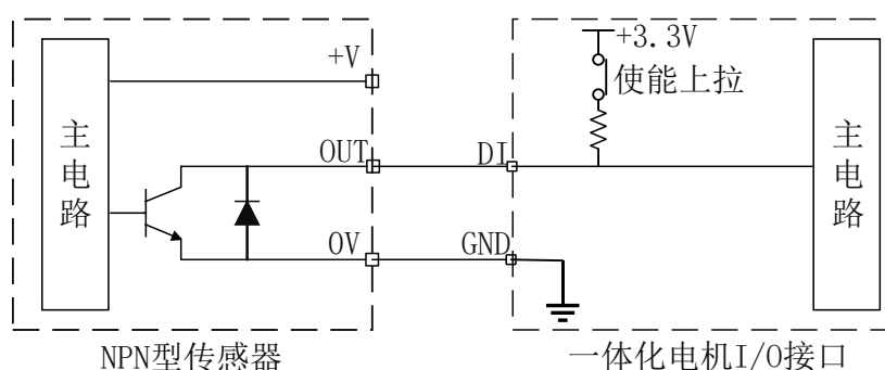
图 3-16 DI 输入端接 NPN 型传感器示意图
