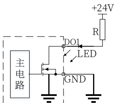
图 3-14 DO1 输出端口接 LED 指示灯示意图
