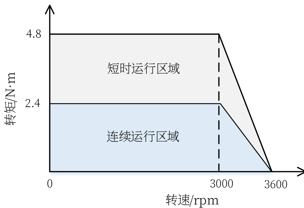
图 2-9 PMMP8075X-COE/CANopen/485-X 矩频特性图 (48V, 18.00A)
