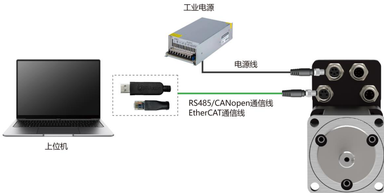
图 4-4 一体化电机调试接线图
