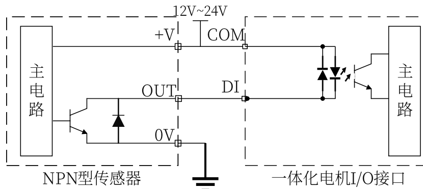
图 3-9 DI 输入端接 NPN 型传感器示意图
