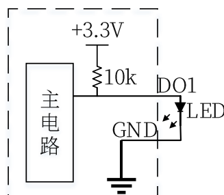
图 3-19 DO 输出端口接 LED 灯示意图
