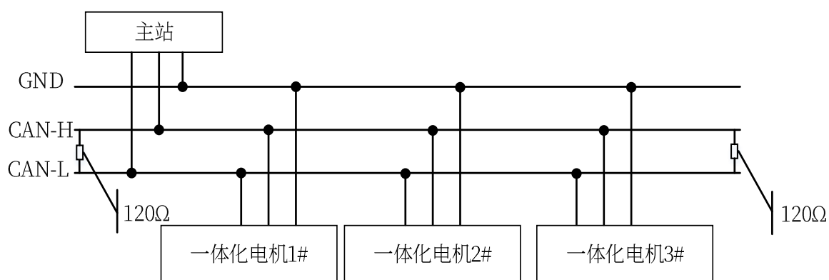
图 4-2 CANopen 通信接线示意图
