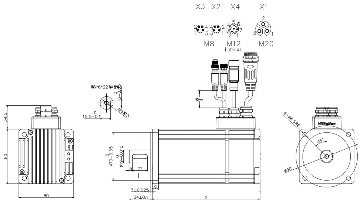
图 2-4 PMMP80 系列一体化电机结构图
