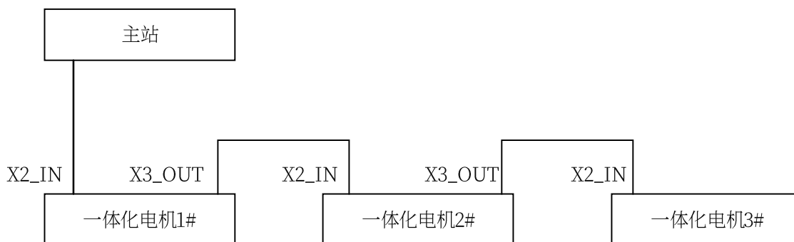
图 4-1 EtherCAT 通信接线示意图
