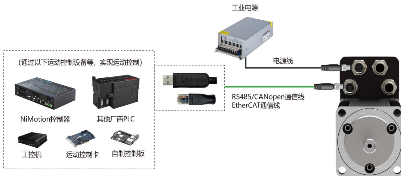
图 4-5 外部控制接线图（通过通信总线控制）
