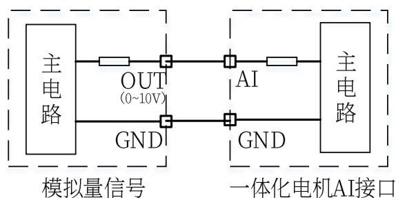
图 3-20 AI 端口接模拟量输入示意图
