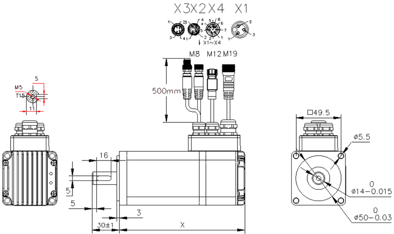
图 2-3 PMMP60 系列一体化电机结构图
