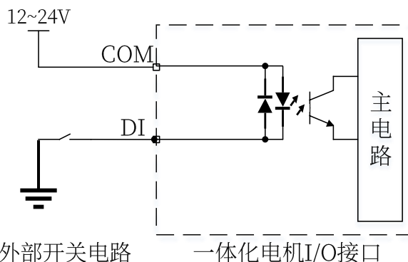
图 3-11 DI 输入端接开关示意图（共阳极）
