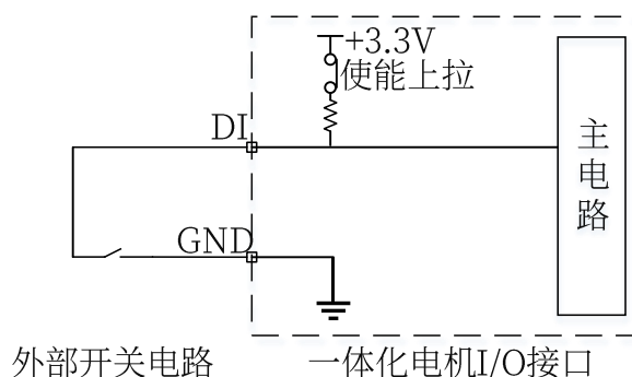
图 3-18 DI 输入端接开关示意图
