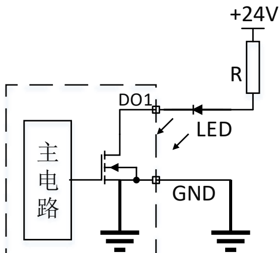
图 3-8 DO 输出端口接 LED 指示灯示意图
