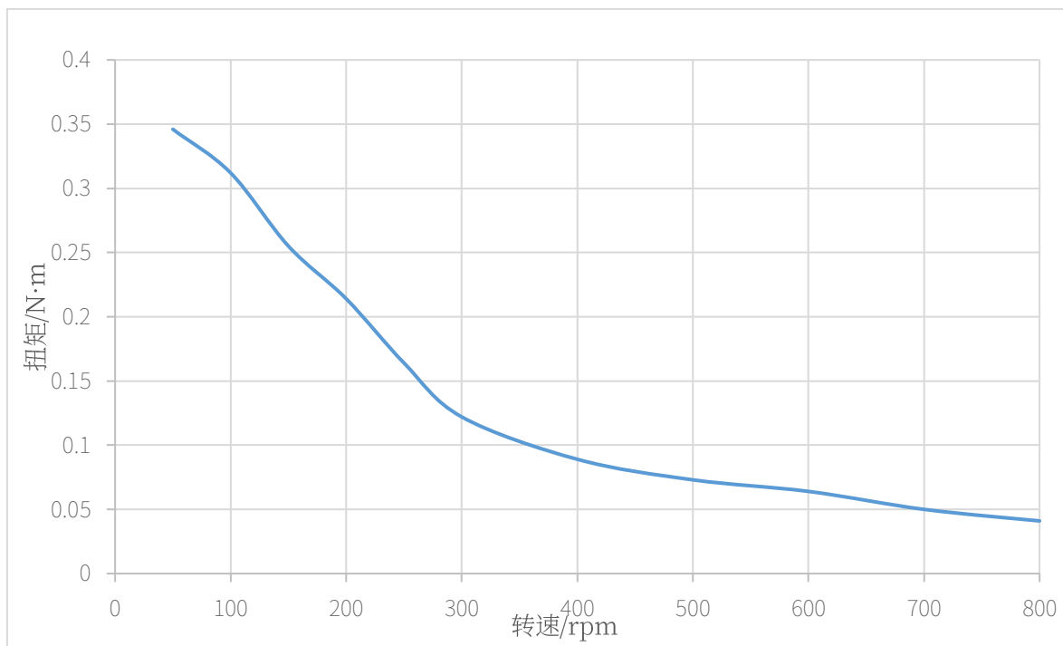
图 2-5 STM3548X-CANopen/485-MC-XX 矩频特性图 (24V, 1.0A)
