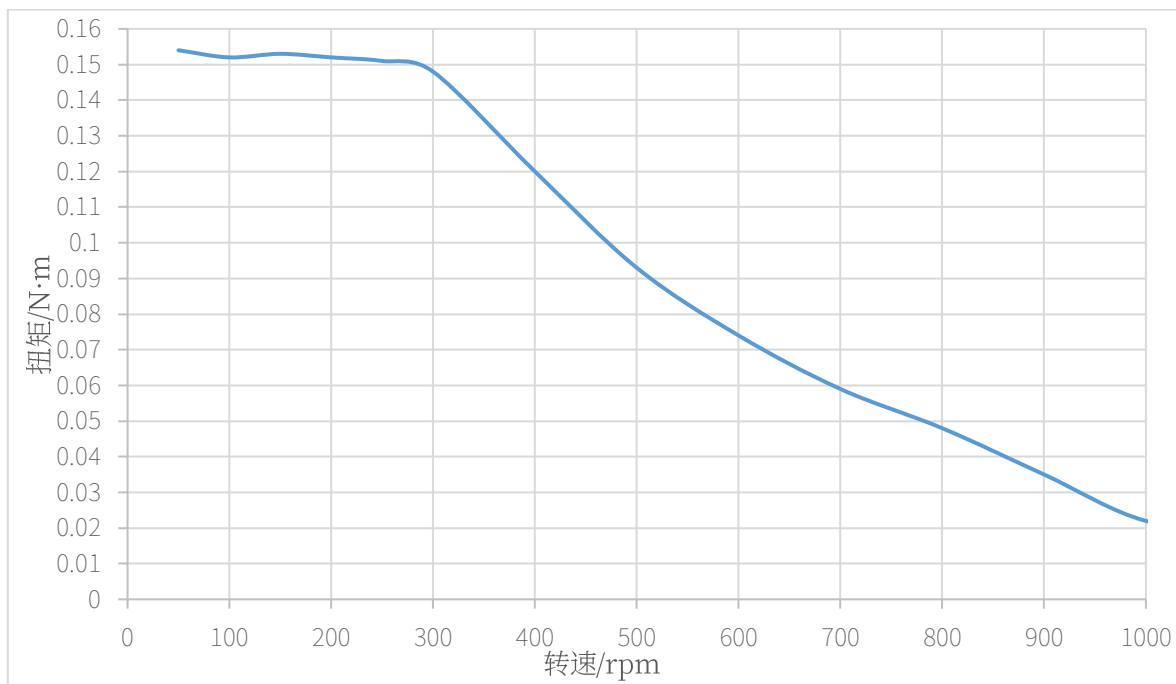
图 2-3 STM3528X-CANopen/485-MC-XX 矩频特性图 (24V, 1.0A)
