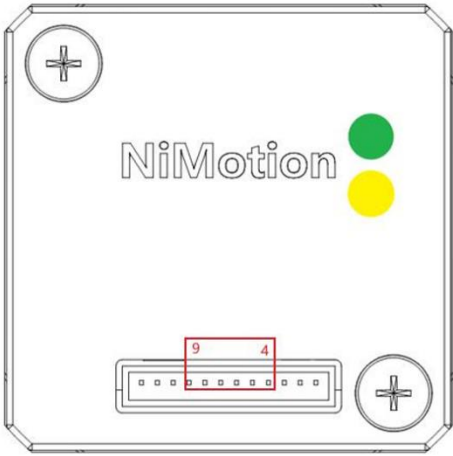
图 3-4 I/O 端口
