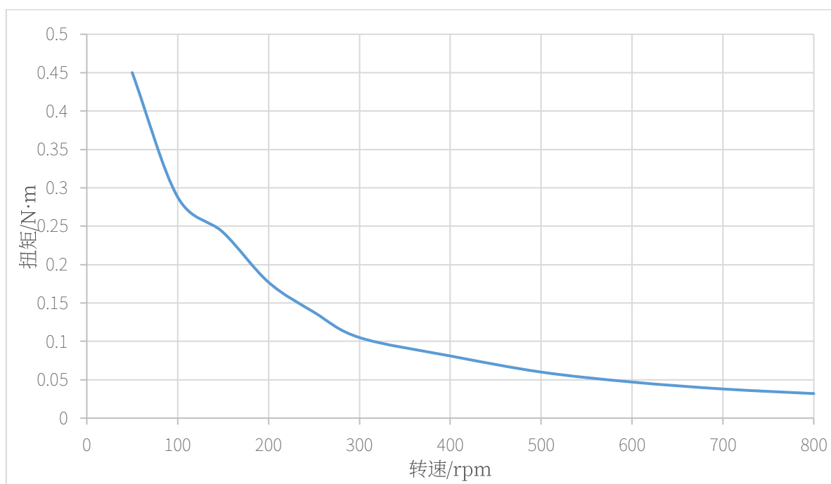
图 2-6 STM3554X-CANopen/485-MC-XX 矩频特性图 (24V, 1.0A)
