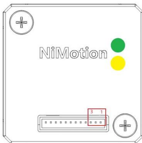
图 3-3 通信端口
