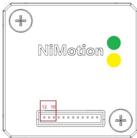
图 3-2 电源端口
