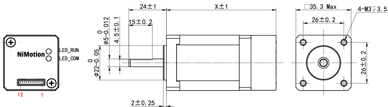
图 2-2 产品整机结构图
