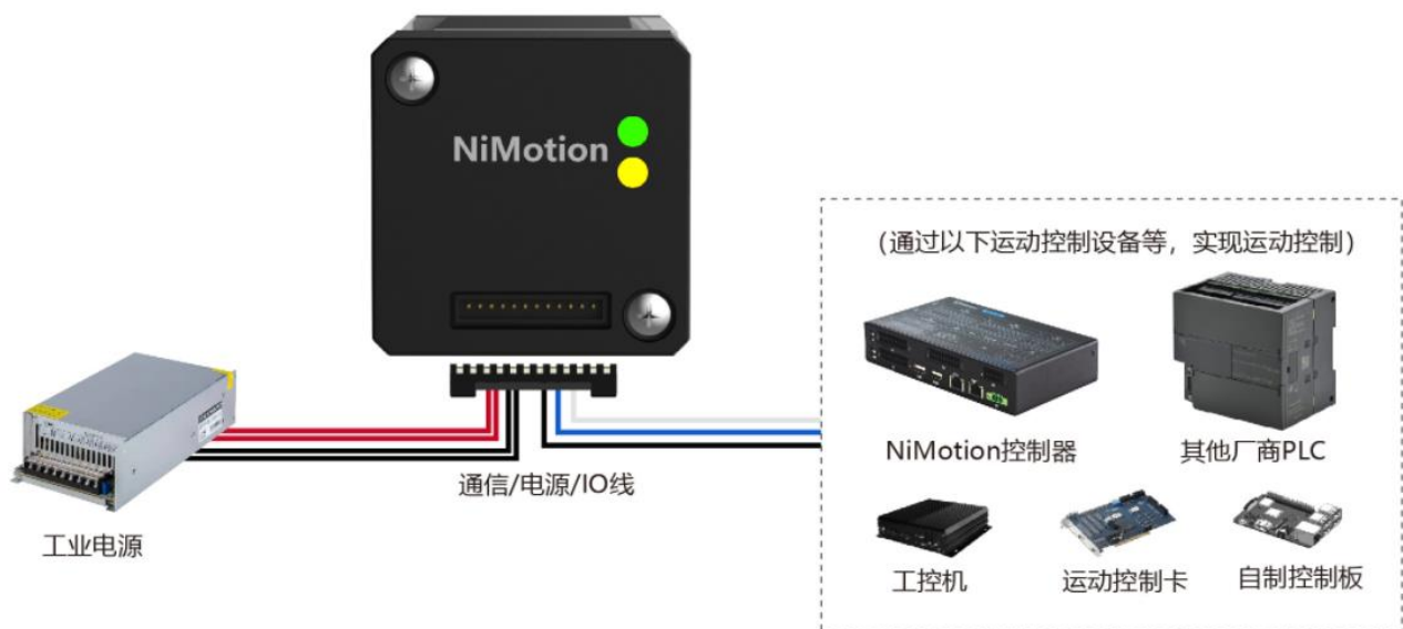
图 4-4 外部控制接线示意图（通过通信总线控制）
