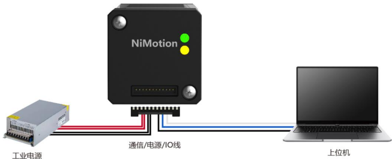
图 4-3 一体化电机调试接线示意图
