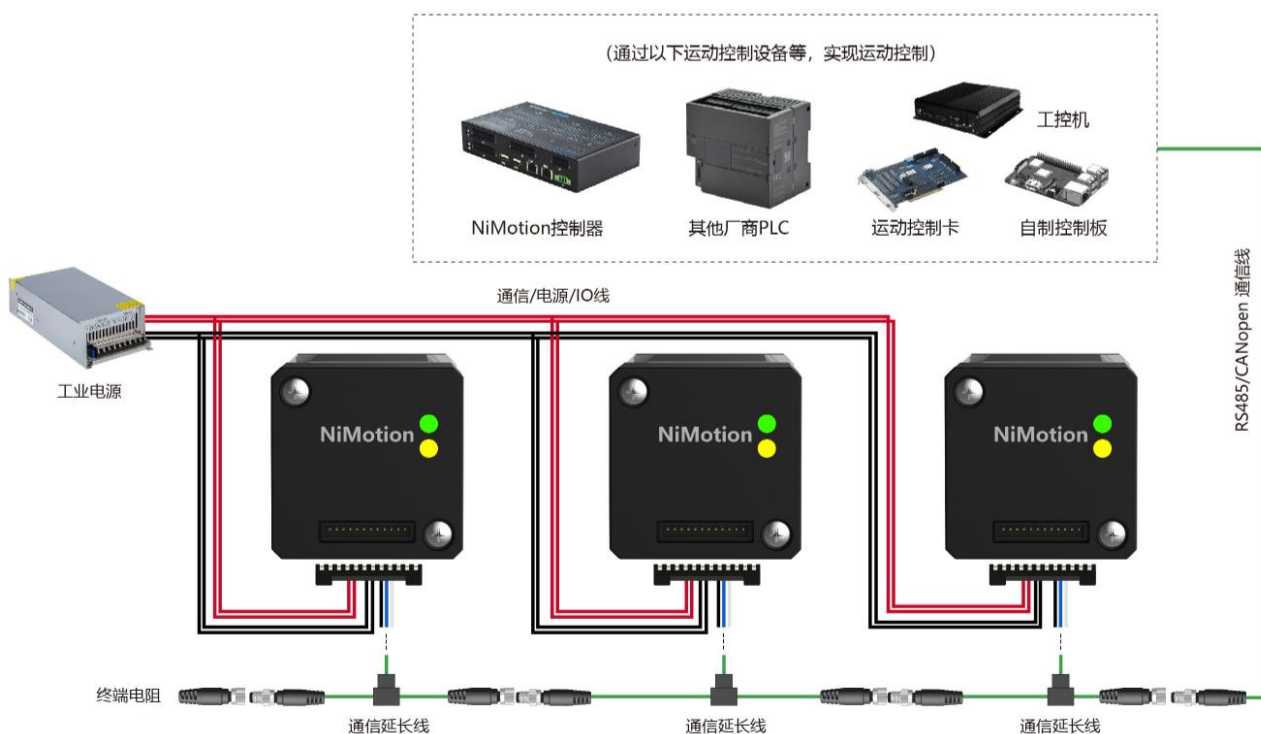
图 4-7 组网接线示意图 (CANopen&RS485)
