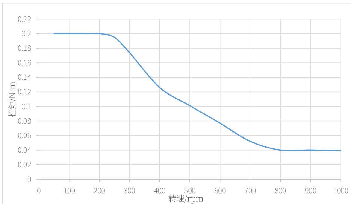
图 2-4 STM3534X-CANopen/485-MC-XX 矩频特性图 (24V, 1.0A)
