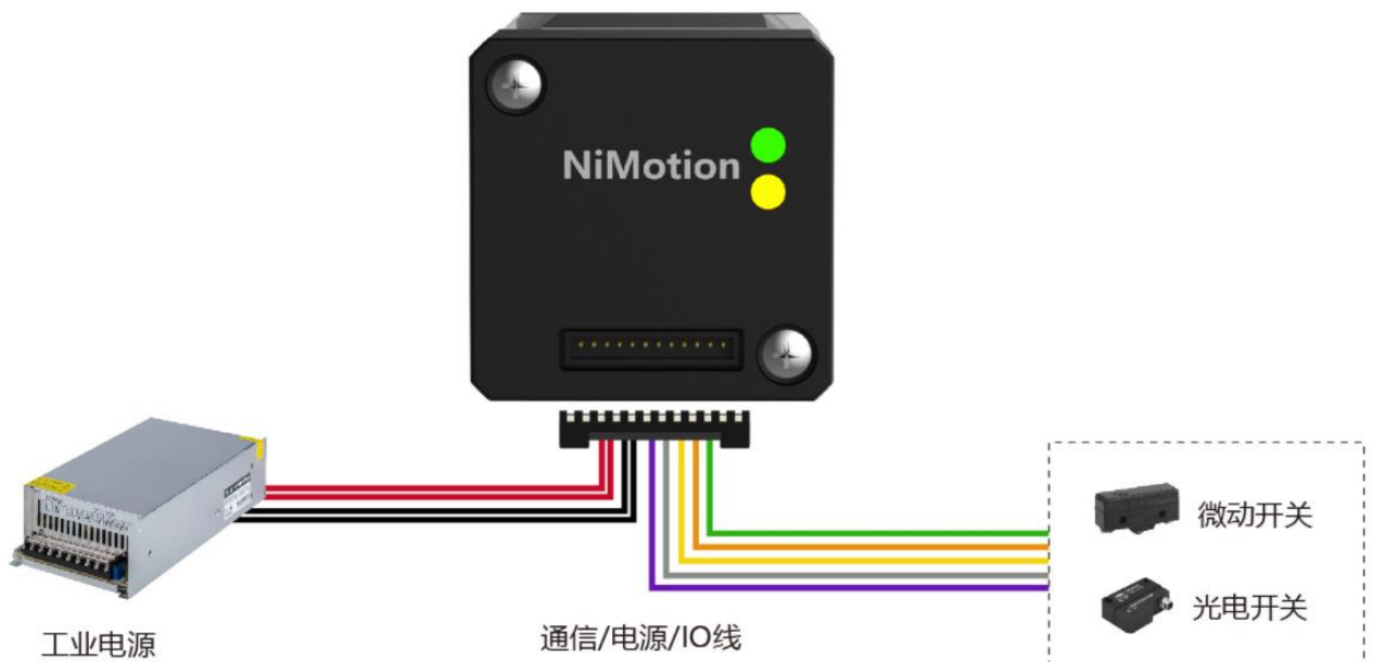
图 4-6 外部控制接线示意图（通过 IO 端口控制）
