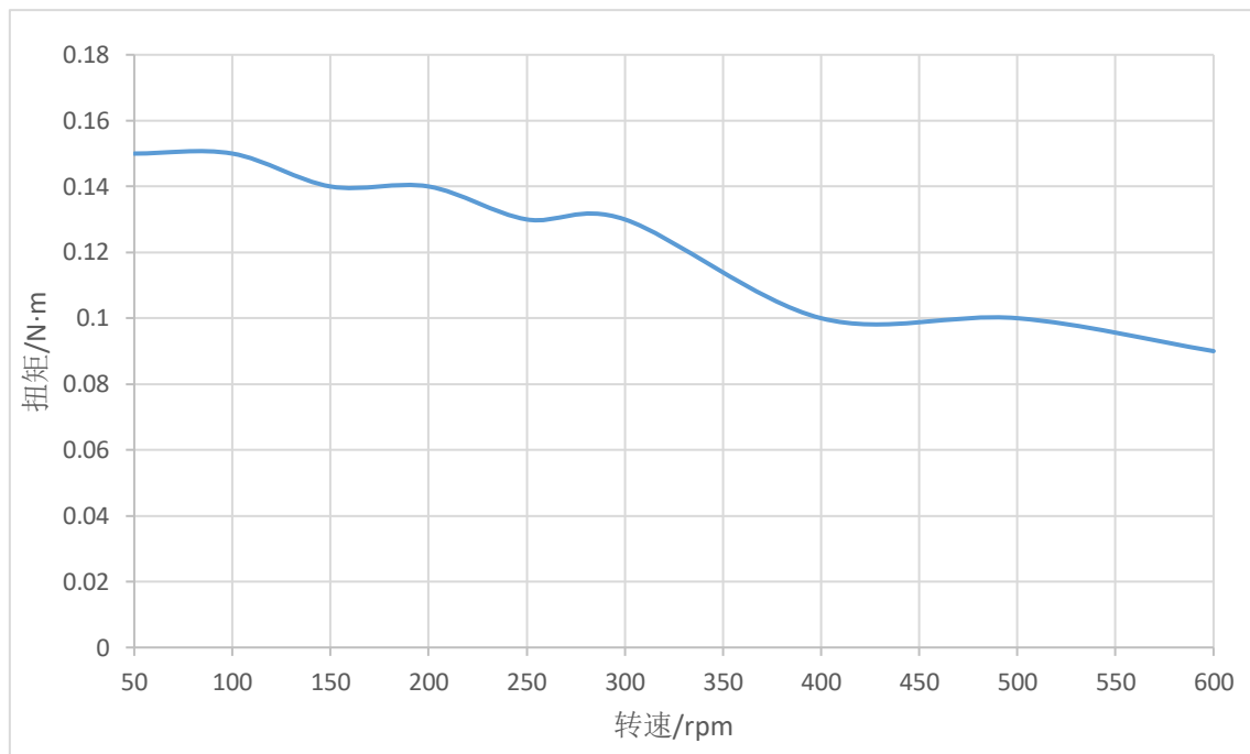
图 4 STM4228A-CAN/485-XX 矩频特性图（24V，0.6A，1/8 细分）
