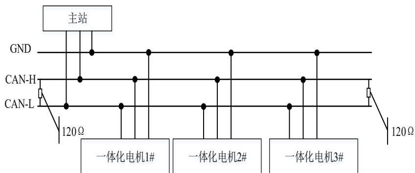
图 14 CAN 通信接线示意图
