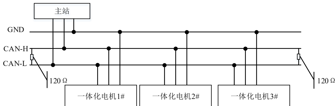
图 19 CANopen 通信接线拓扑图
