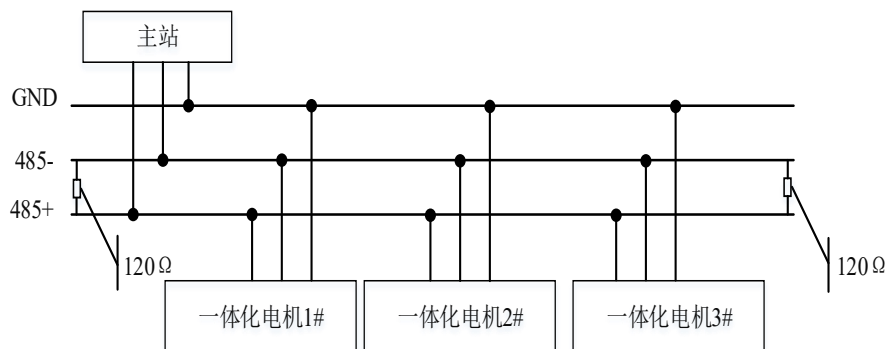
图 13 RS485 通信接线示意图
