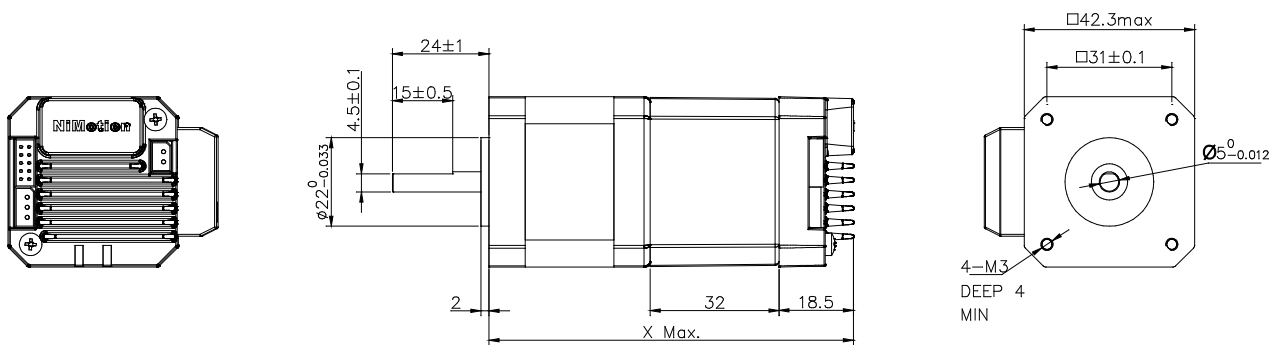
图 3 结构图（制动器款）
