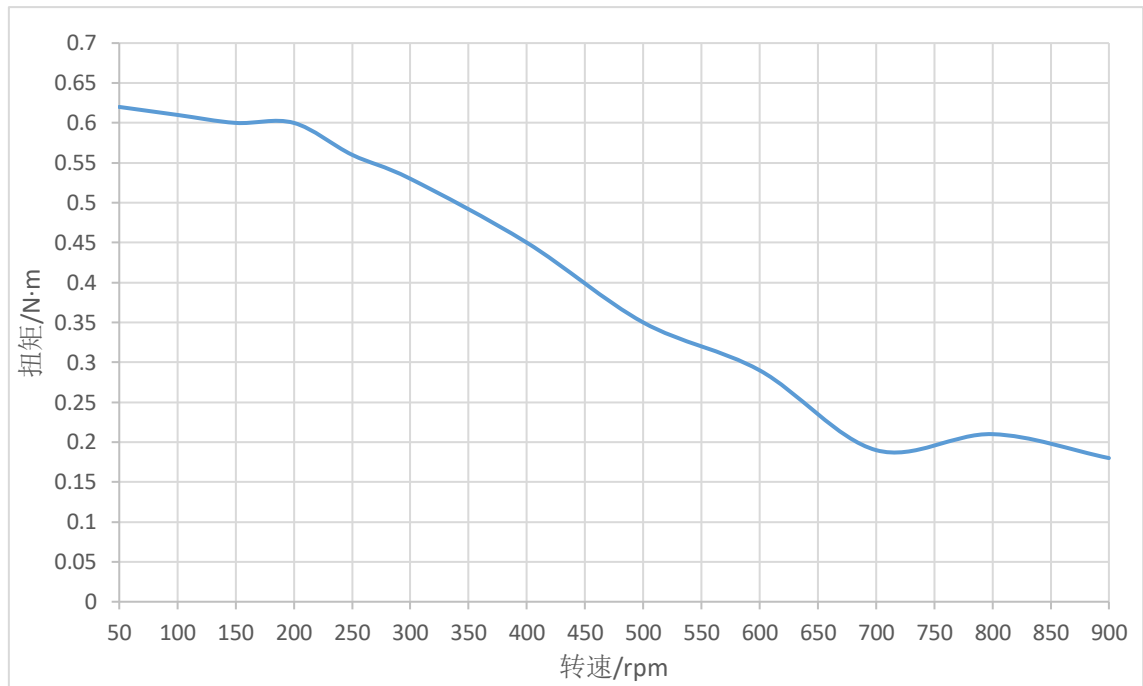
图 8 STM4260A-CAN/485-XX 矩频特性图（24V，2.0A，1/8 细分）
