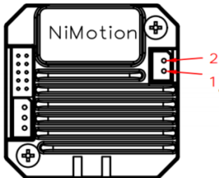
图 10 电源端口
