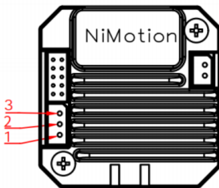
图 11 电机通信端口
