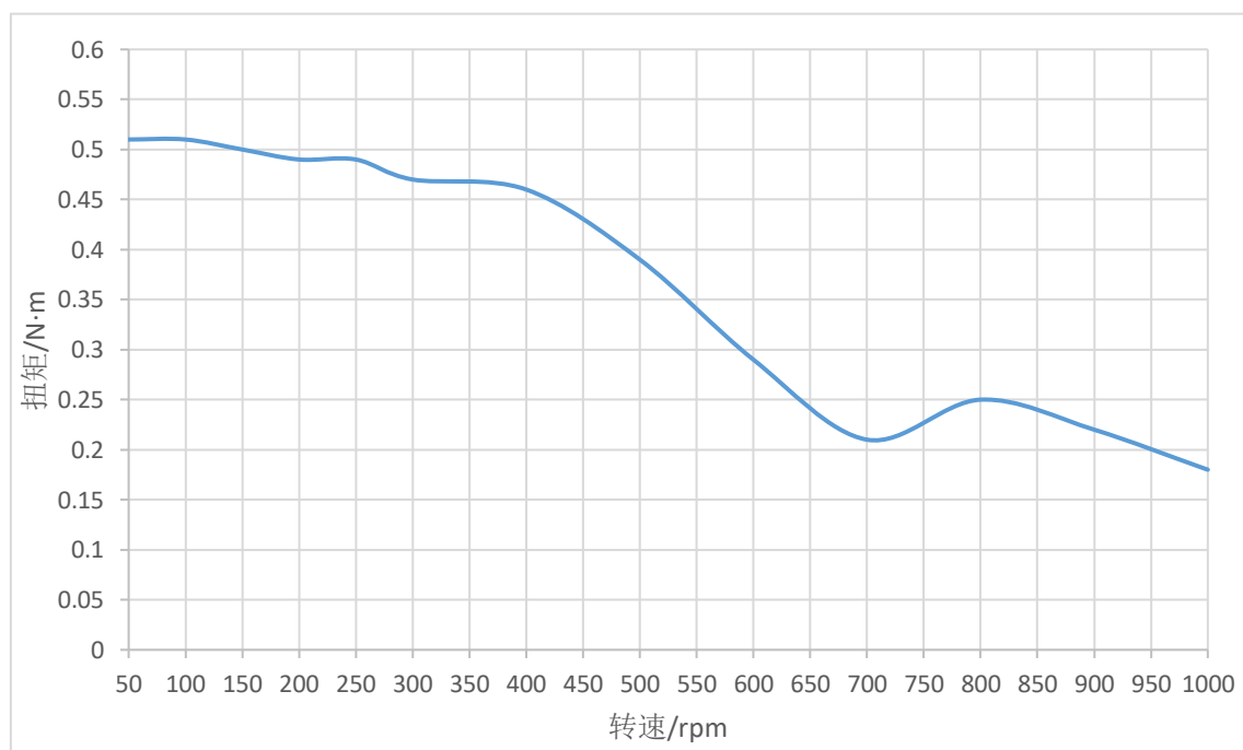
图 7 STM4248A-CAN/485-XX 矩频特性图（24V，1.7A，1/8 细分）
