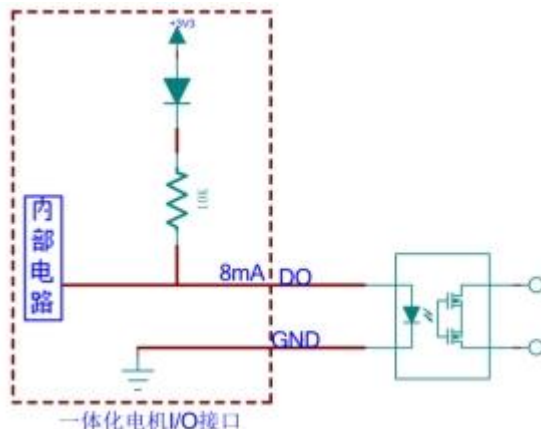
图 17 DO 输出端口接 photoMOS 器件示意图
