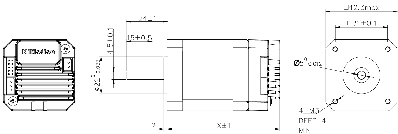
图 2 结构图（标准款）
