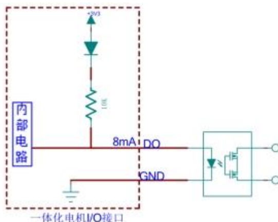
图 16 DO 输出端口接 photoMOS 器件示意图
