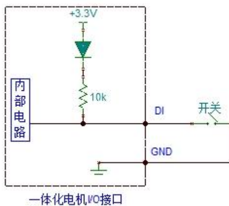
图 15 DI 输入端口接开关示意图
