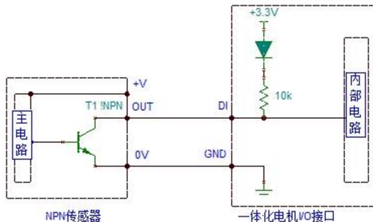
图 14 DI 输入端口接 NPN 传感器示意图
