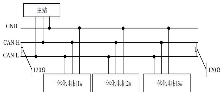
图 13 CANopen 通信接线示意图
