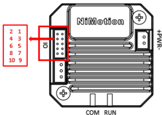
图 12 I/O 输入输出端口
