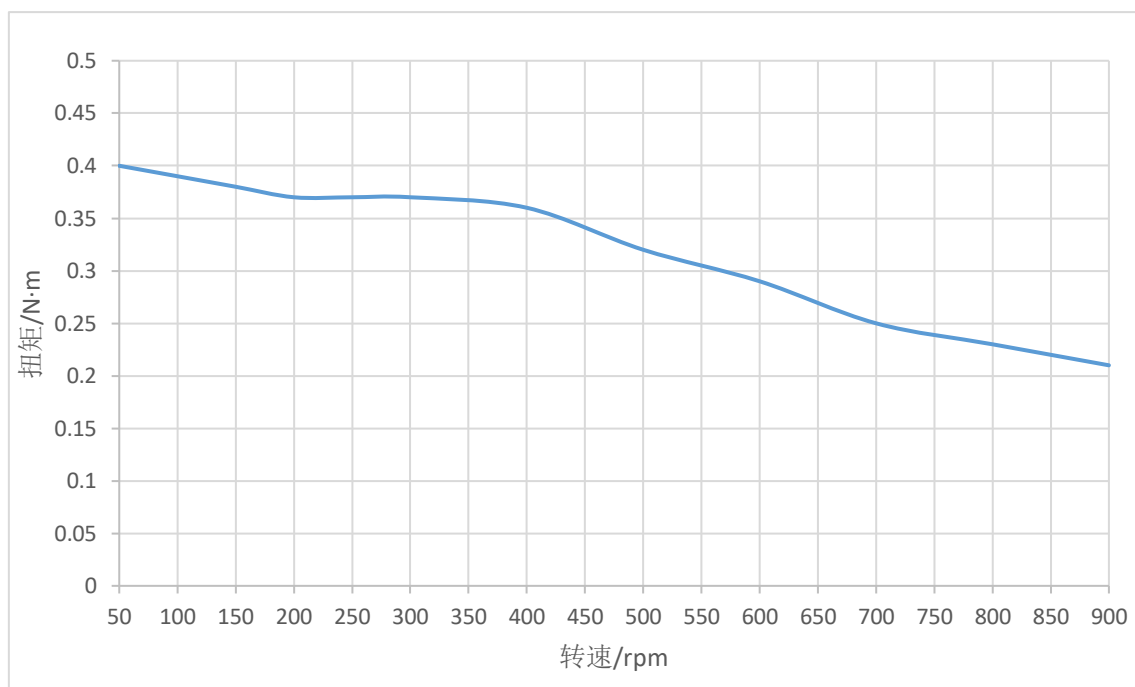
图 6 STM4240(A)-CANopen-XX 矩频特性图（24V，1.7A，1/8 细分）
