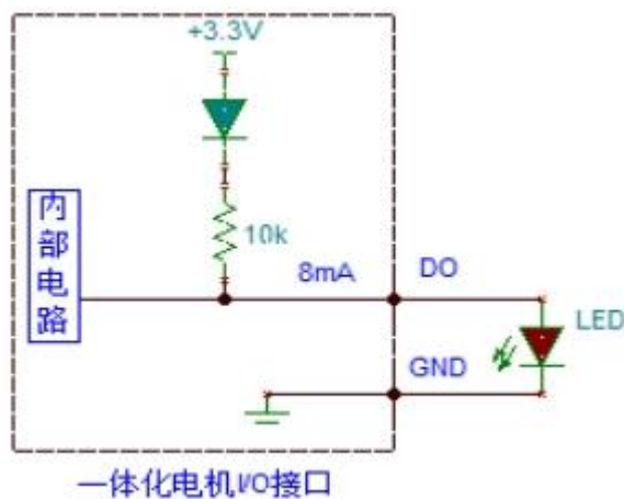
图 17 DO 输出端口接 LED 灯示意图
