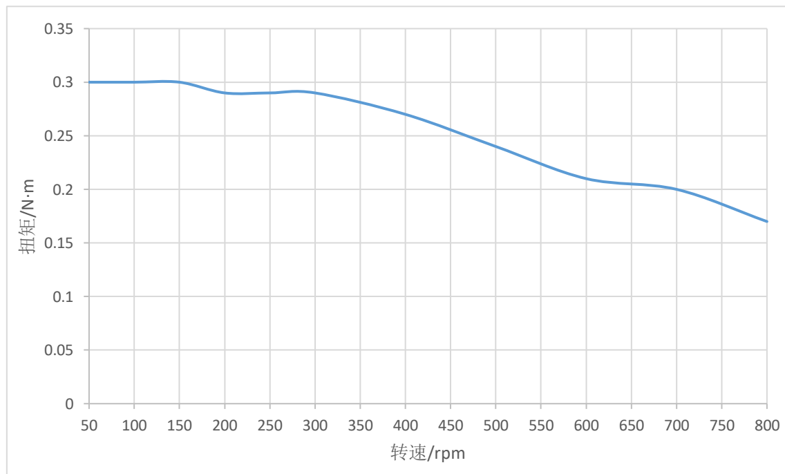
图 5 STM4234(A)-CANopen-XX 矩频特性图（24V，1.3A，1/8 细分）
