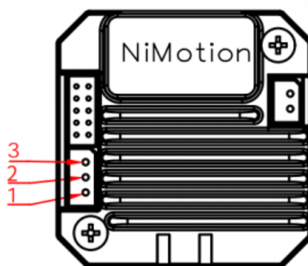
图 11 通信端口
