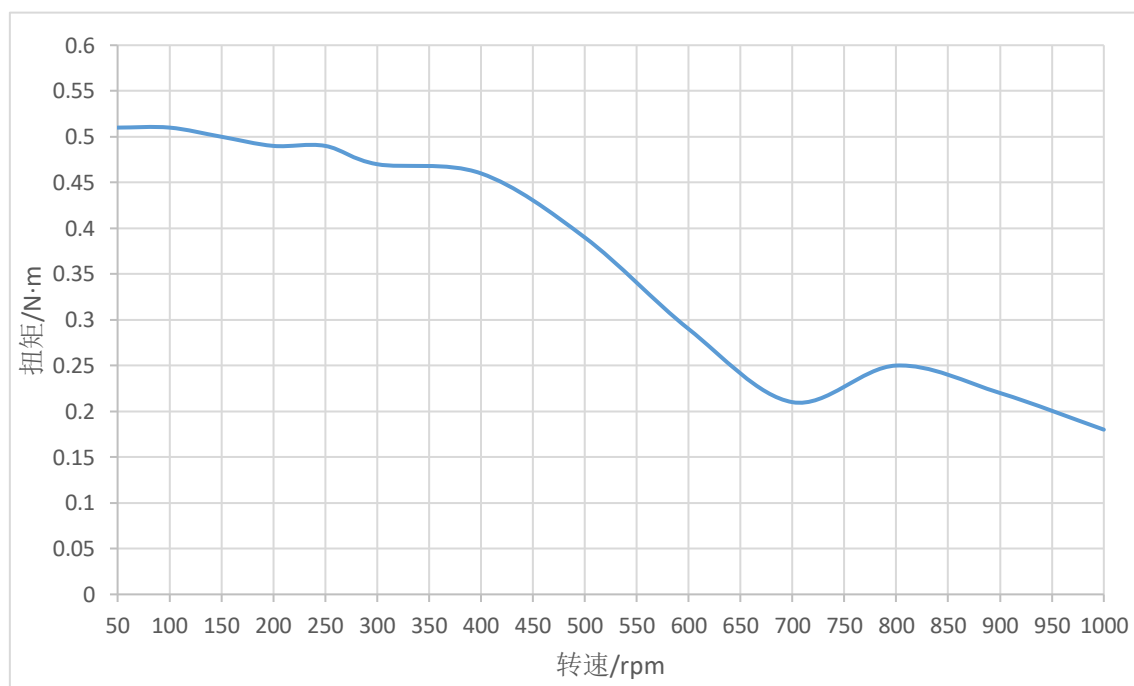
图 7 STM4248(A)-CANopen-XX 矩频特性图（24V，1.7A，1/8 细分）
