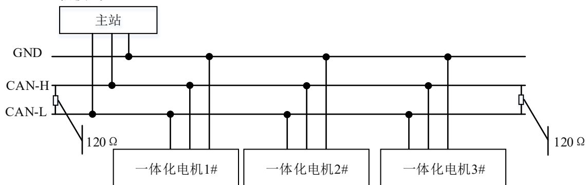
图 18 CANopen 通信接线拓扑图
