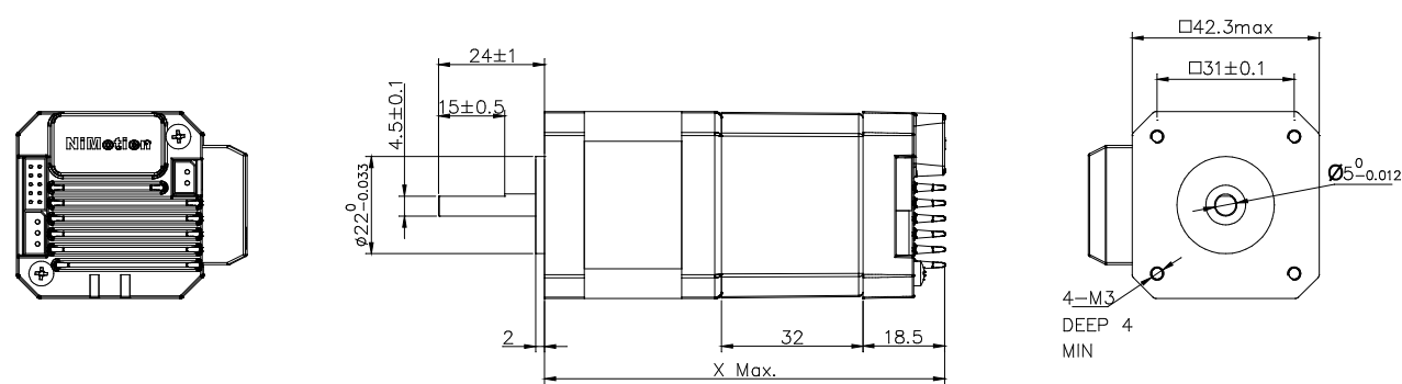
图 3 结构图（制动器款）
