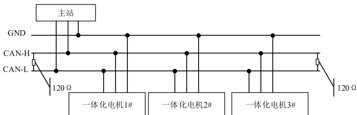
图 4-1 CANopen 通信接线拓扑图
