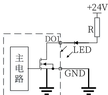
图 3-9 DO1 输出端口接 LED 指示灯示意图
