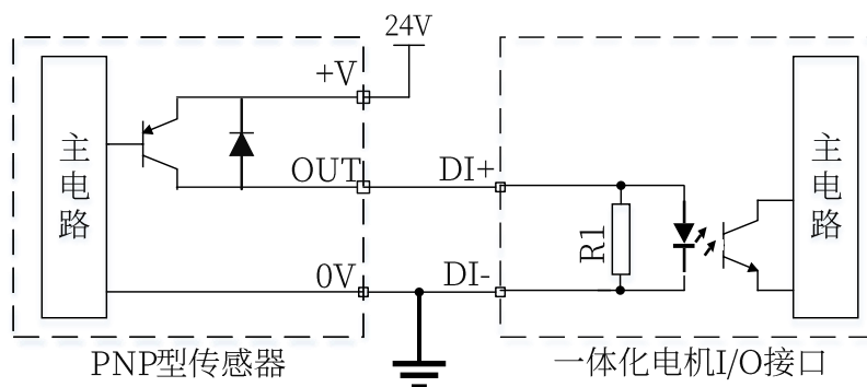
图 3-6 DI 输入端口接 PNP 型传感器示意图
