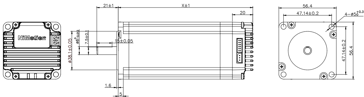
图 2-2 产品整机结构图（标准款）
