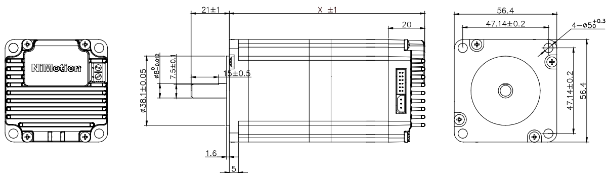
图 2-4 产品整机结构图（制动器款）
