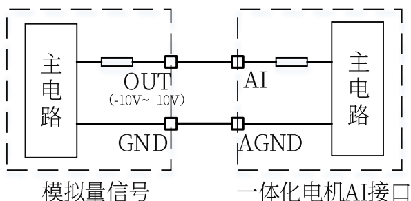
图 3-11 AI 端口接模拟量输入示意图
