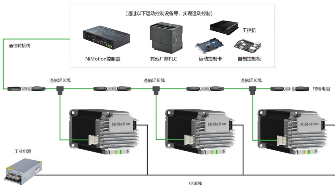
图 4-7 组网接线图 (CANopen&RS485)
