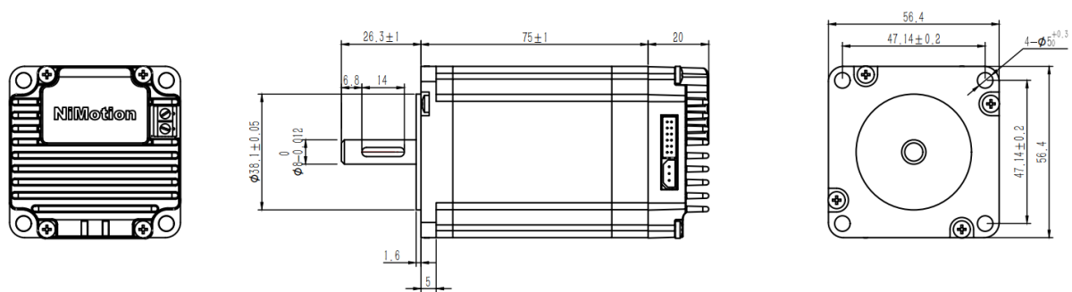
图 2-3 STM5776B-XXX-1FH 产品整机结构图
