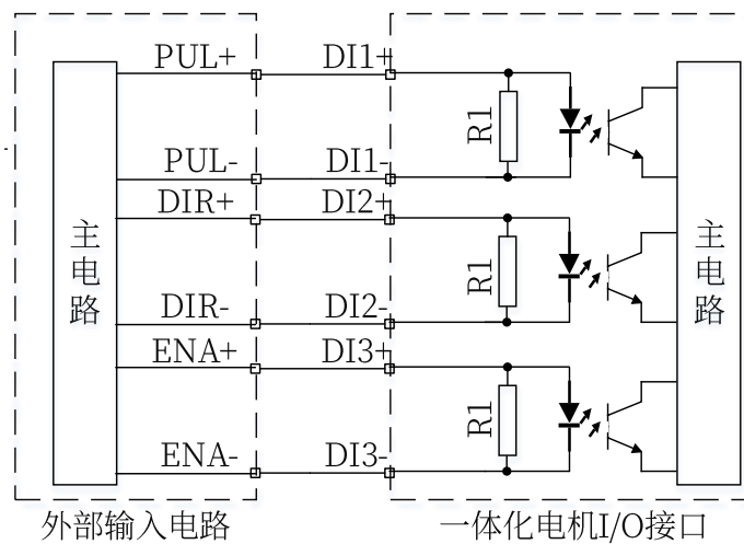
图 3-8 DI 输入端口接脉冲输入示意图
