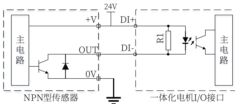
图 3-5 DI 输入端口接 NPN 型传感器示意图
