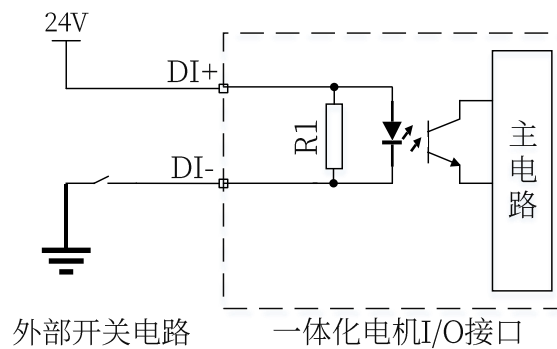
图 3-7 DI 输入端口接开关示意图
