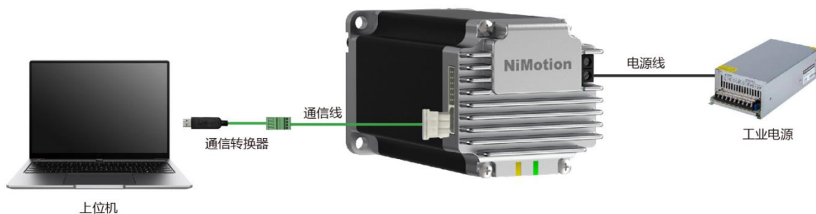
图 4-3 一体化电机调试接线图
