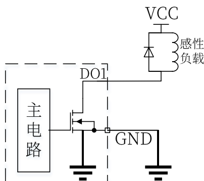
图 3-10 DO 输出端口接感性负载示意图
