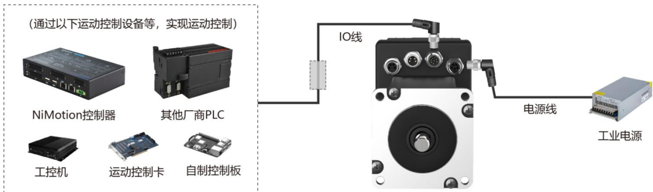
图 4-5 外部控制接线图
