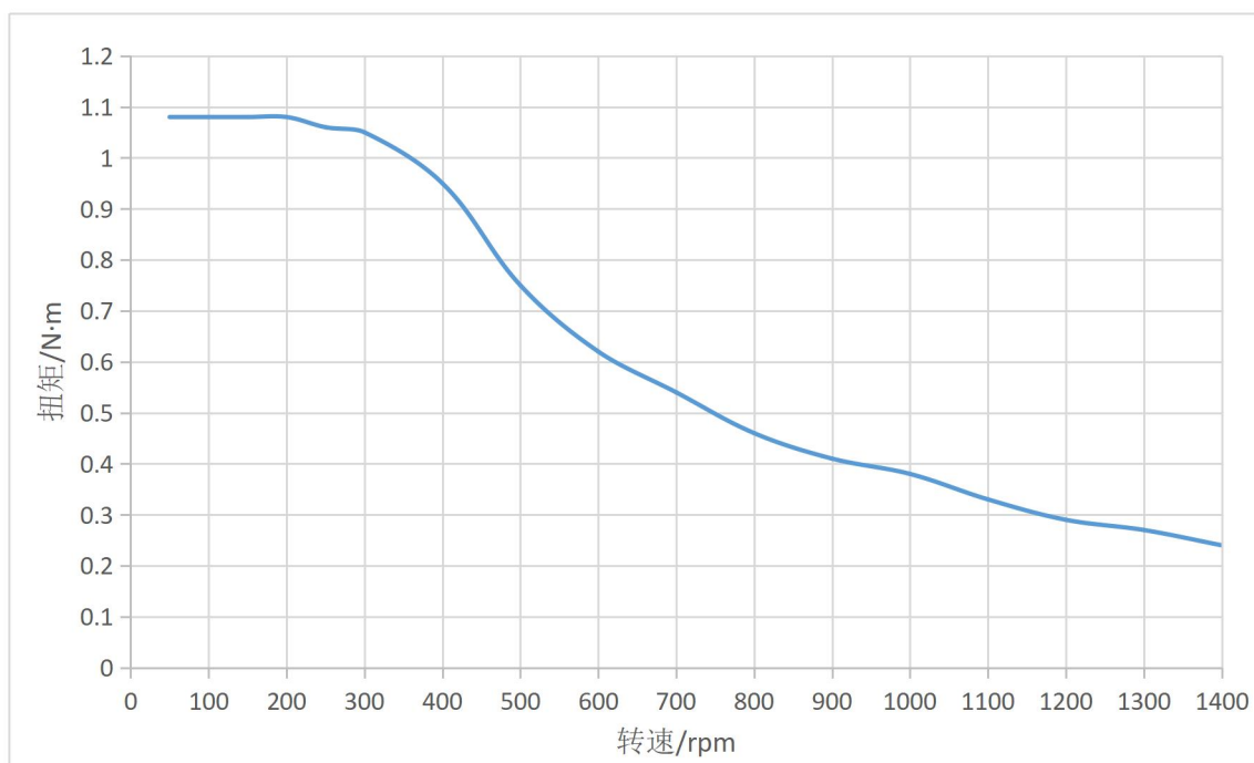
图 2-3 STMPW5756X-XX 矩频特性图（48V，3.0A）
