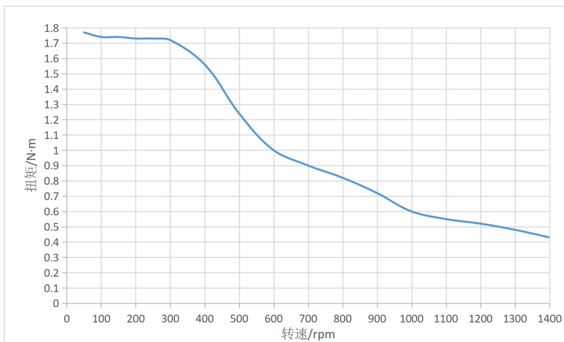
图 2-4 STMPW5776X-XX 矩频特性图（48V，4.2A）
