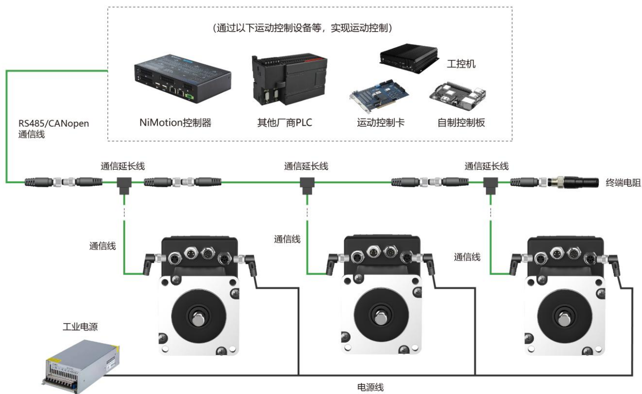
图 4-7 通信组网接线图
