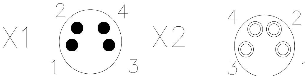
图 3-3 通信端口
