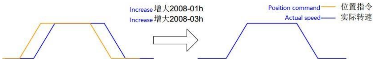
图 7-3 位置环增益
