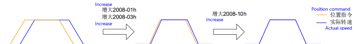
图 7-5 速度前馈
