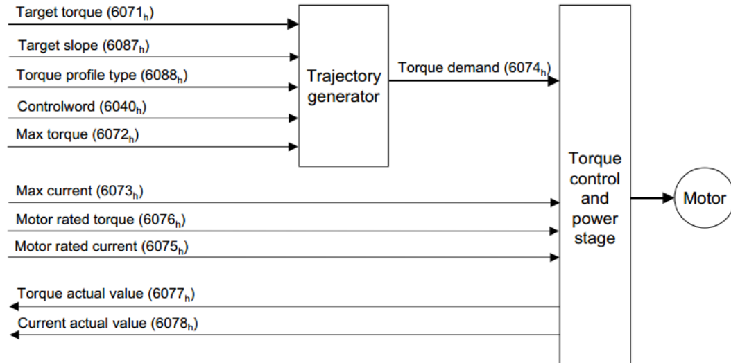
图 5-17 控制框图
