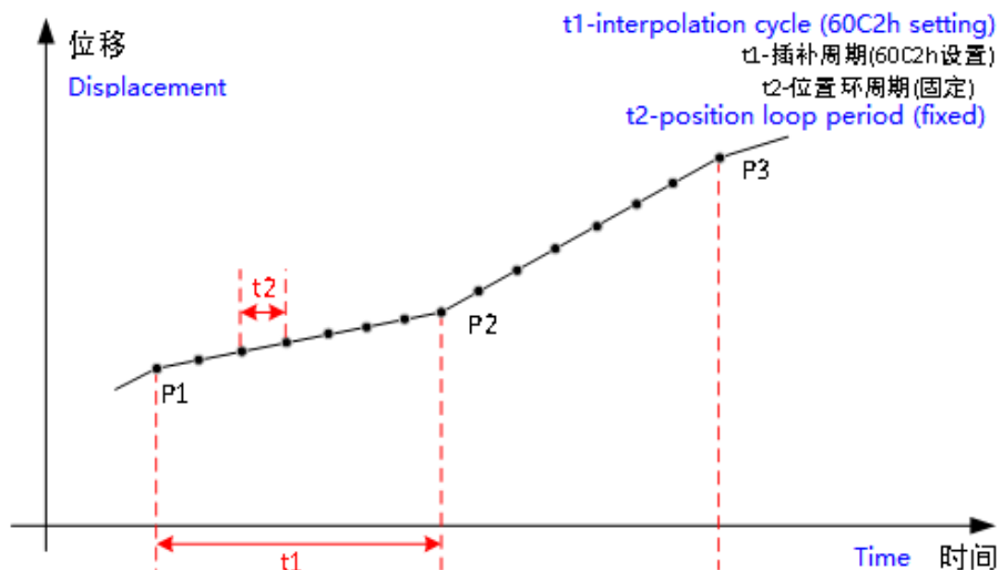
图 5-21 插补示意图
