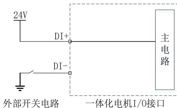
图 3-7 DI 输入端口接开关示意图
