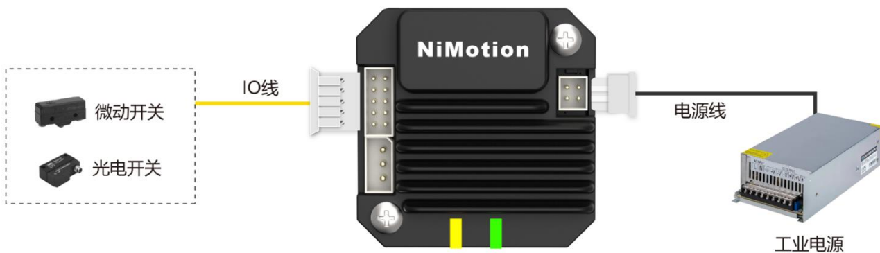
图 4-6 外部控制接线图
