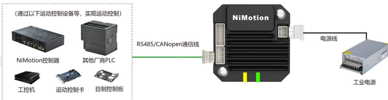
图 4-4 外部控制接线图（通过通信总线控制）
