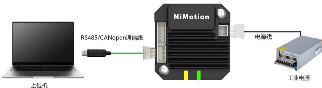
图 4-3 一体化电机调试接线图
