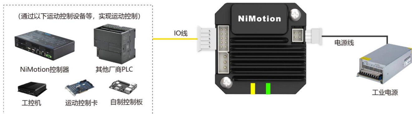
图 4-5 外部控制接线图
