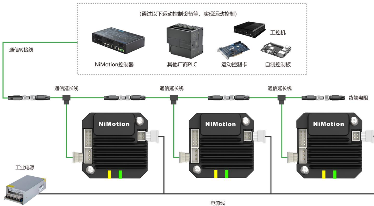
图 4-7 RS485&CANopen 通信组网接线图
