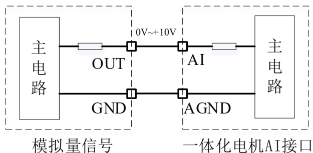
图 3-9 AI 端口接模拟量输入示意图
