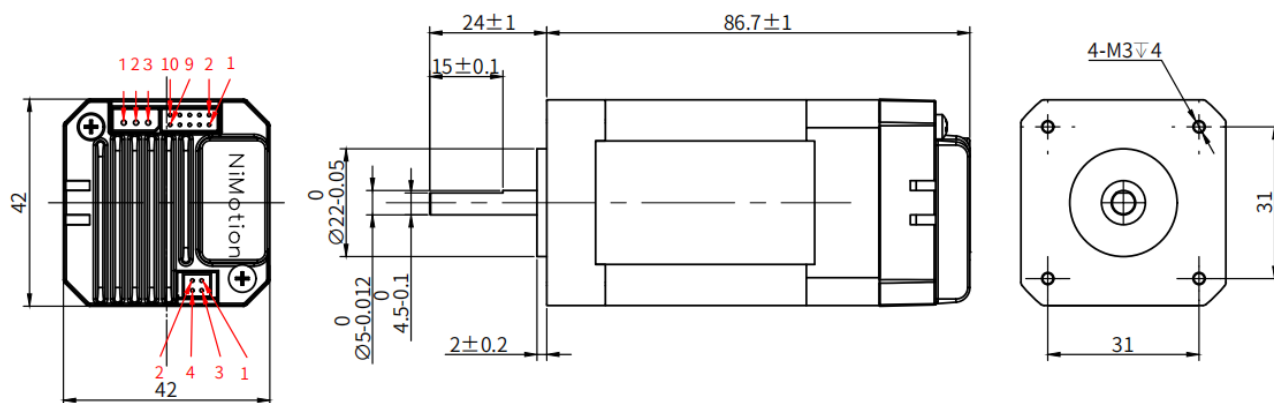
图 2-2 产品结构图
