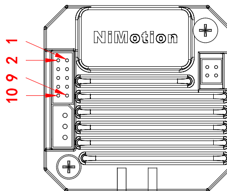
图 3-4 I/O 输入输出端口
