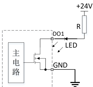
图 3-8 DO1 输出端口接 LED 指示灯示意图
