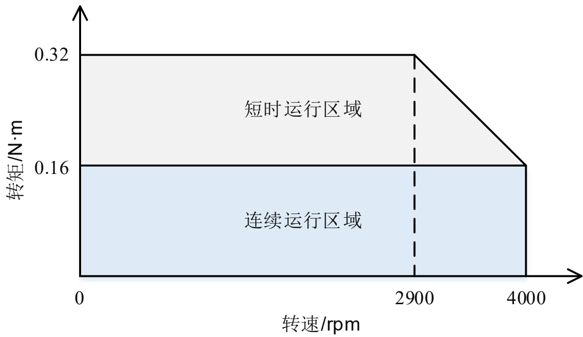
图 2-3 BLM4206B-CANopen/485-N-XX 矩频特性图 (24V, 4.0A)
