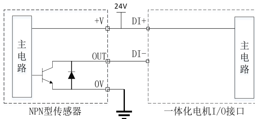
图 3-5 DI 输入端口接 NPN 型传感器示意图
