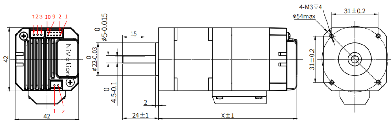
图 2-4 结构图 (制动器款)
