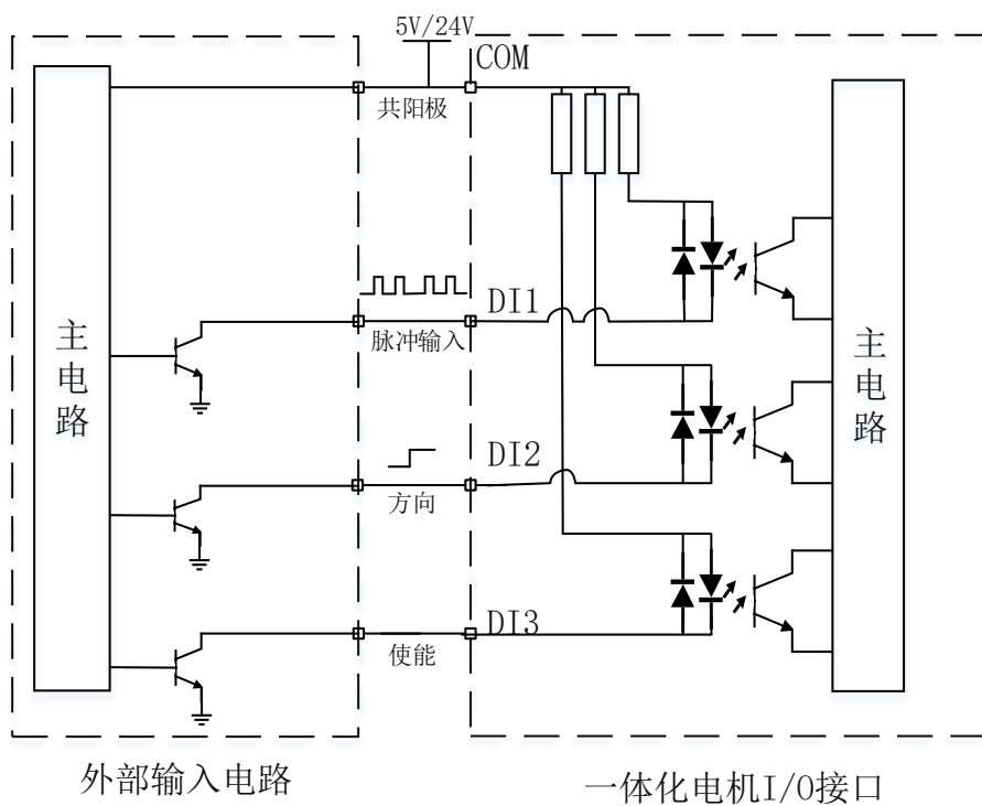
图 3-8 DI 输入端口接脉冲输入示意图
