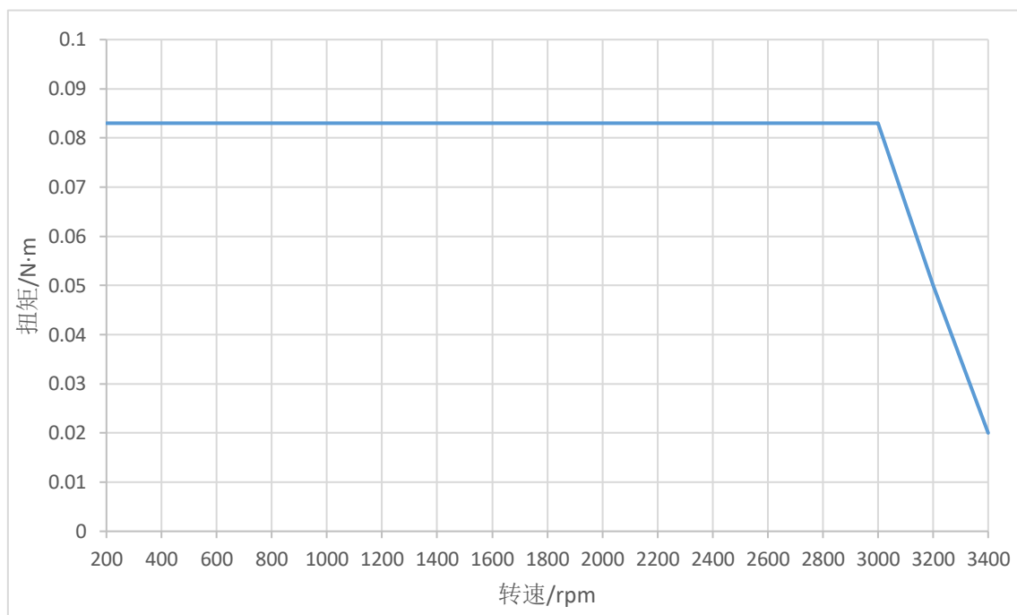
图 2-5 BLM4203B-CANopen/485-XX 矩频特性图 (24V, 1.7A)
