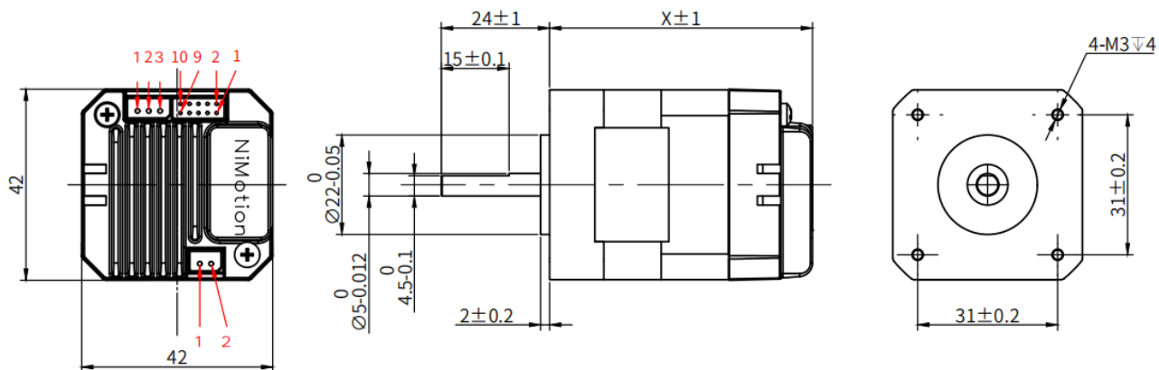
图 2-2 结构图(标准款, 内出线)
