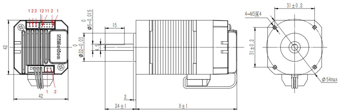
图 2-3 结构图(标准款, 外出线)
