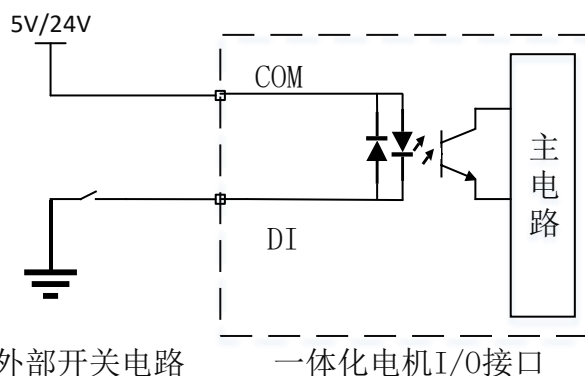
图 3-6 DI 输入端口接开关示意图（共阳极）
