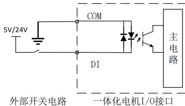
图 3-7 DI 输入端口接开关示意图（共阴极）
