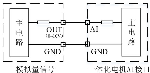
图 3-10 AI 端口接模拟量输入示意图
