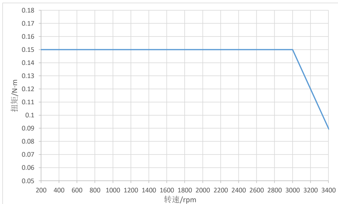
图 2-6 BLM4205-CANopen/485-XX 矩频特性图 (24V, 2.77A)
