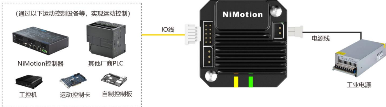
图 4-5 外部控制接线图
