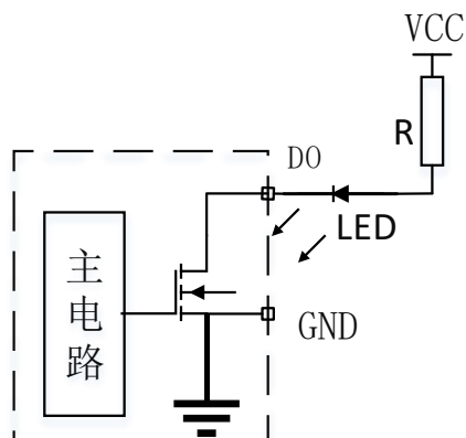
图 3-9 DO1 输出端口接 LED 指示灯示意图
