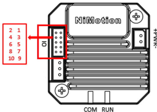
图 3-4 I/O 输入输出端口
