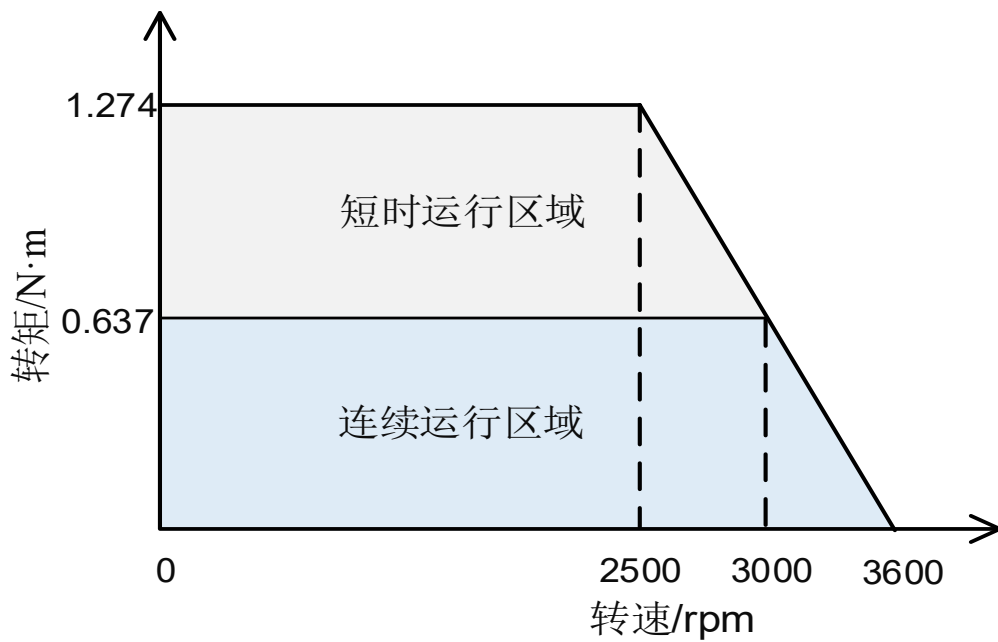
图 2-3 PMM6020B-XXX-LE-XX 矩频特性图 (48V, 6.5A)
