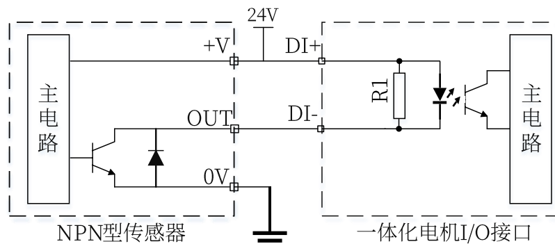
图 3-5 DI 输入端口接 NPN 传感器示意图
