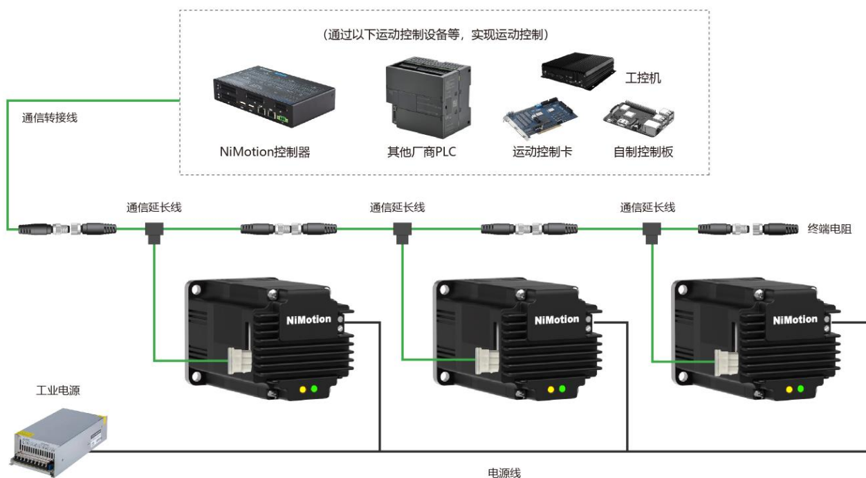
图 4-7 组网接线图 (CANopen&RS485)
