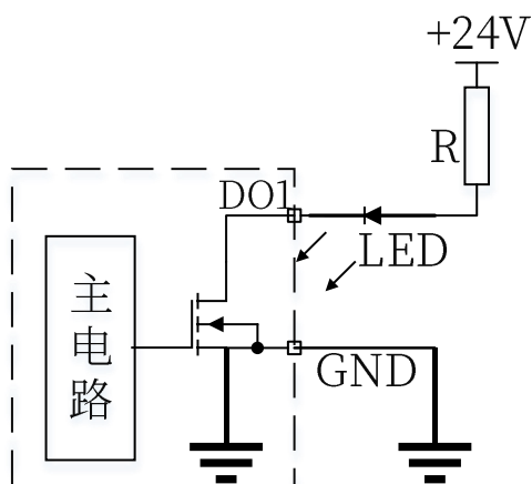
图 3-9 DO 输出端口接 LED 指示灯示意图
