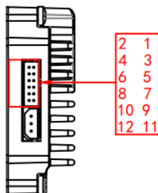
图 3-4 数字量输入输出 (I/O)
