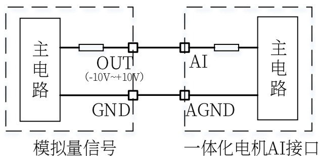
图 3-11 AI 端口接模拟量输入示意图
