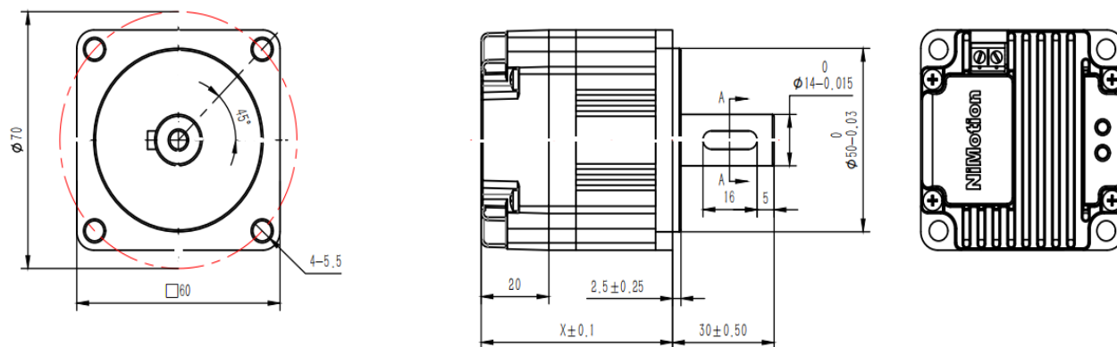
图 2-2 产品整机结构图
