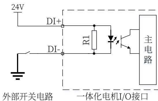
图 3-7 DI 输入端口接开关示意图
