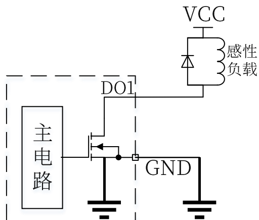
图 3-10 DO 输出端口接感性负载示意图
