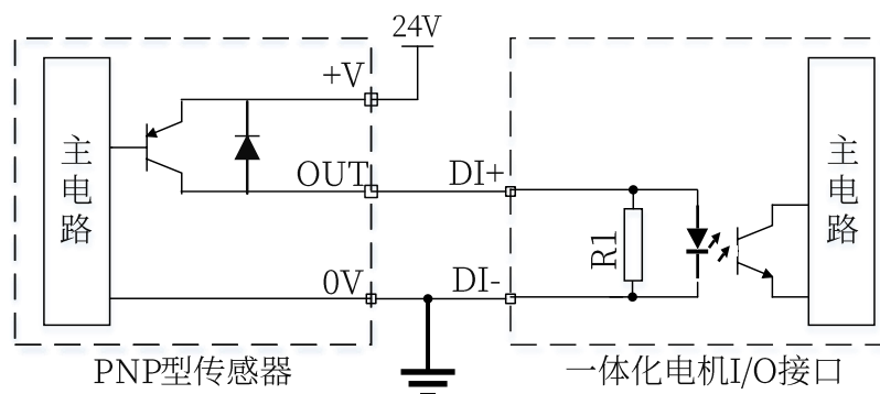
图 3-6 DI 输入端口接 PNP 传感器示意图
