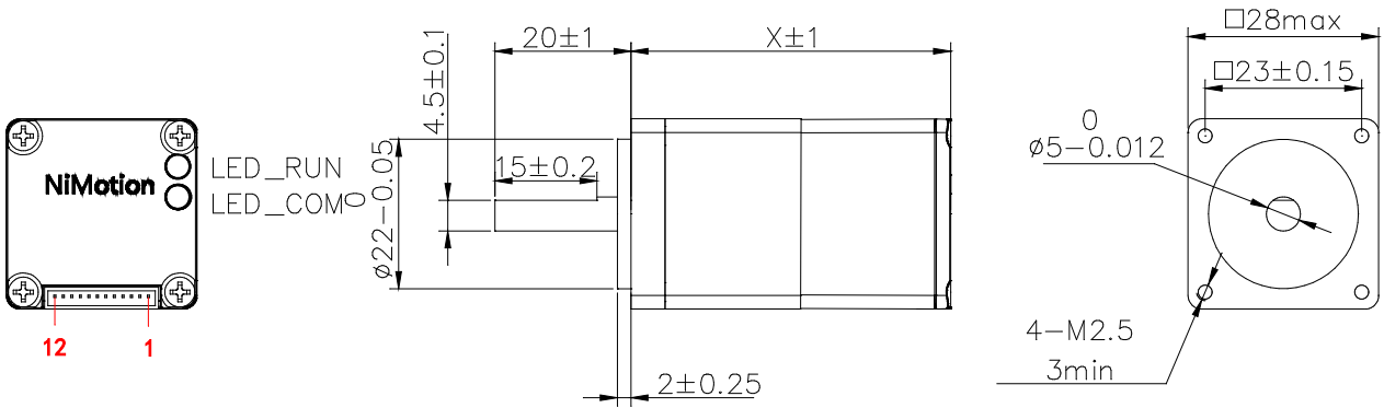
图 2-2 产品整机结构图
