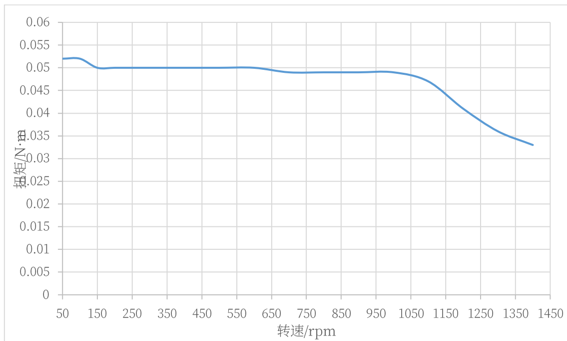
图 2-3 STM2832X-CANopen/485-M-XX 矩频特性图 (24V, 1.0A)
