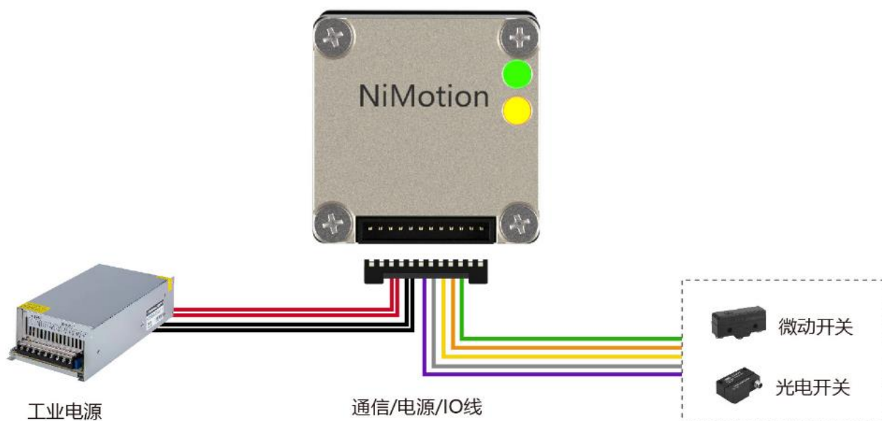
图 4-6 外部控制接线图（通过 IO 端口控制）
