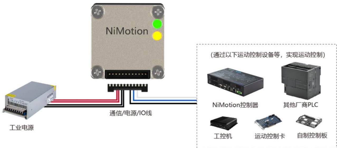
图 4-4 外部控制接线图（通过通信总线控制）
