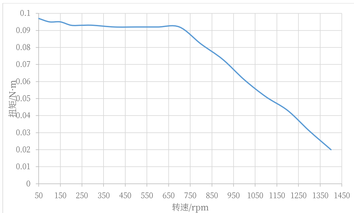
图 2-4 STM2851X-CANopen/485-M-XX 矩频特性图 (24V, 1.0A)
