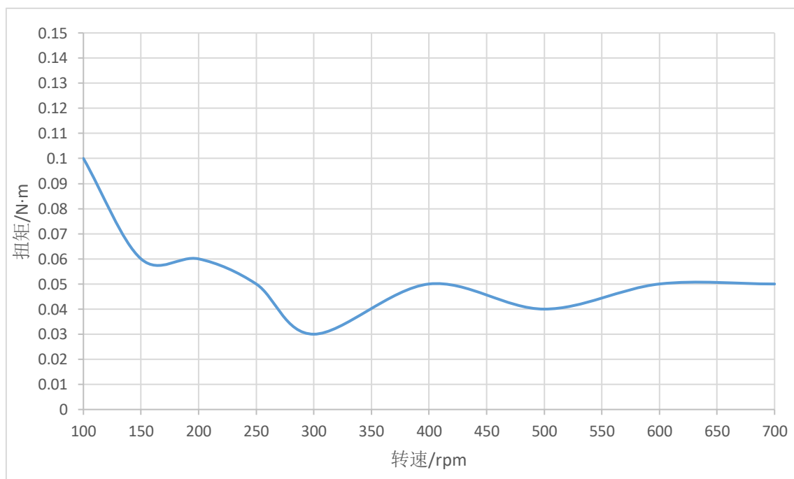
图 4 STM2851A-CANopen-XX 矩频特性图（24V，1.0A，1/8 细分）
