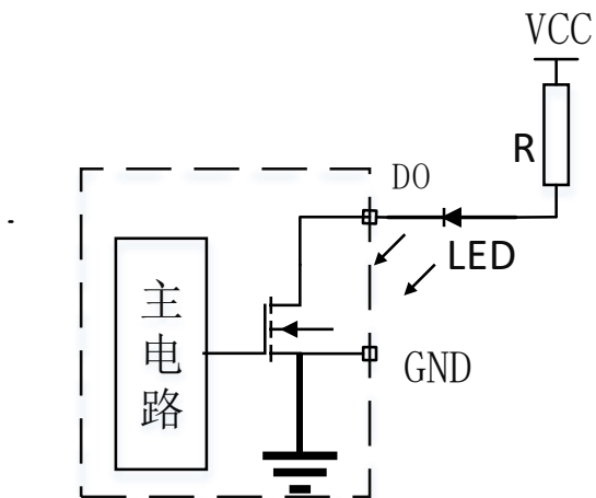
图 12 DO 输出端口接 LED 指示灯示意图
