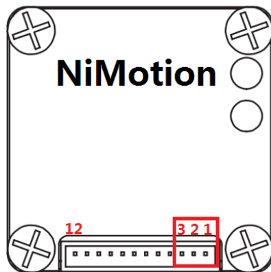
图 7 通信线引脚图
