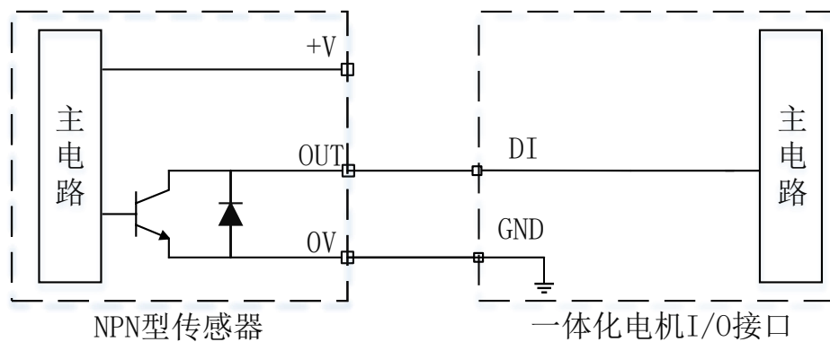
图 10 DI 输入端口接 NPN 型传感器示意图
