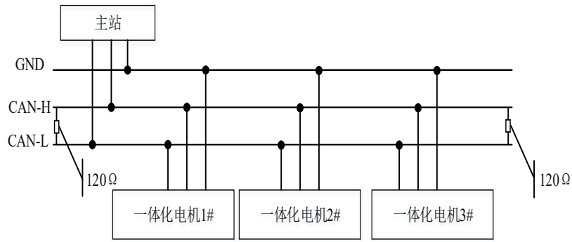
图 9 CANopen 通信接线示意图
