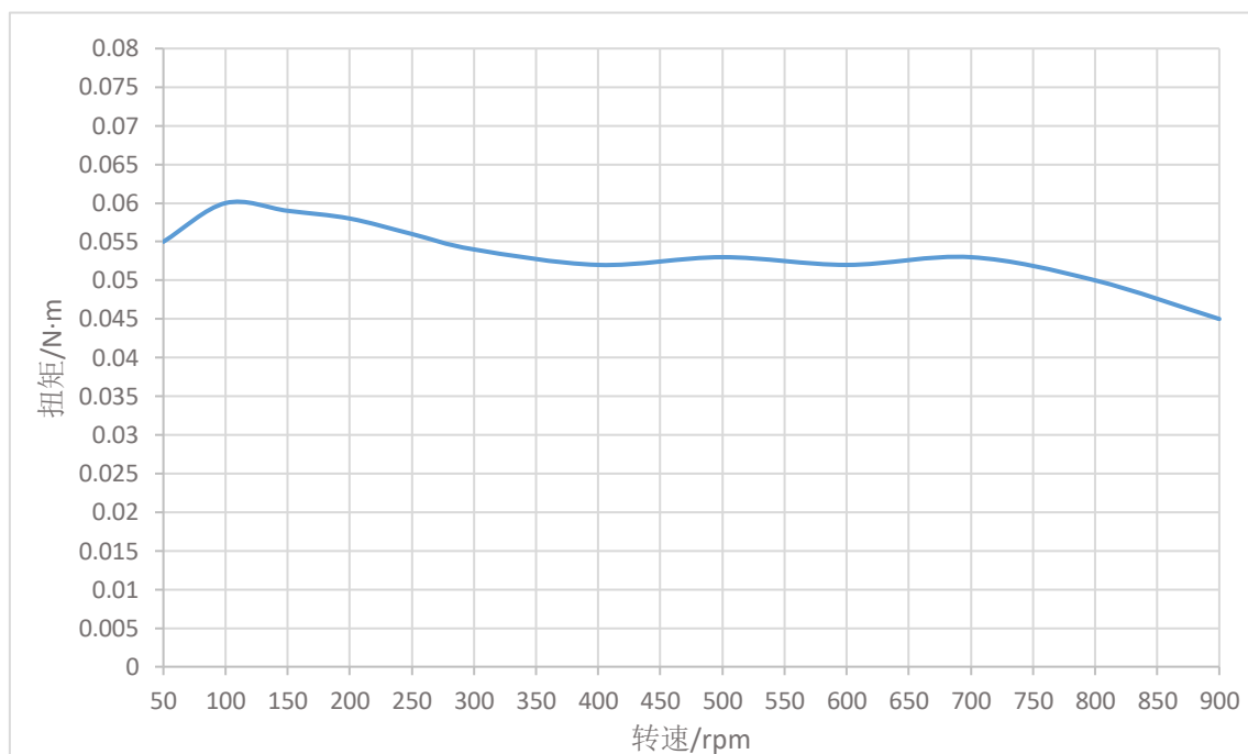
图 3 STM2832A-CANopen-XX 矩频特性图（24V，1.0A，1/8 细分）
