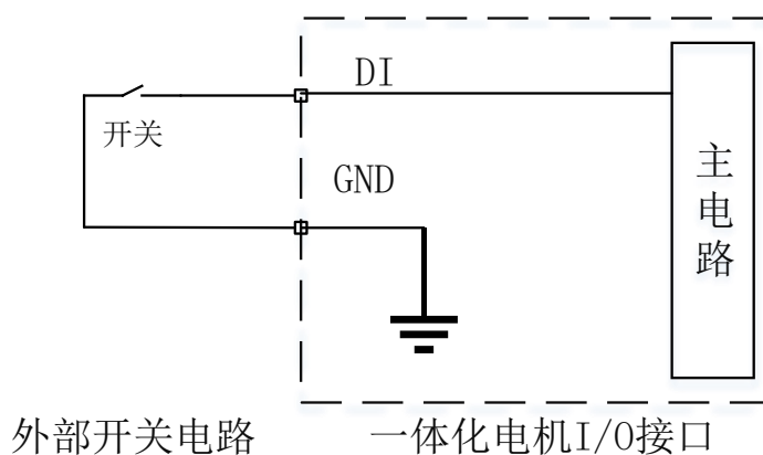
图 11 DI 输入端口接开关示意图
