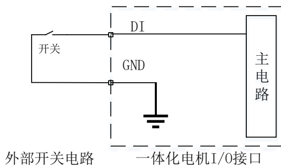
图 13 DI 输入端口接开关示意图
