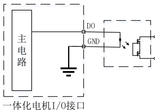
图 14 DO 输出端口接 photoMOS 器件示意图
