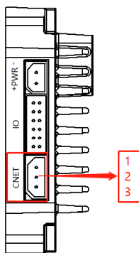
图 9 通信端口
