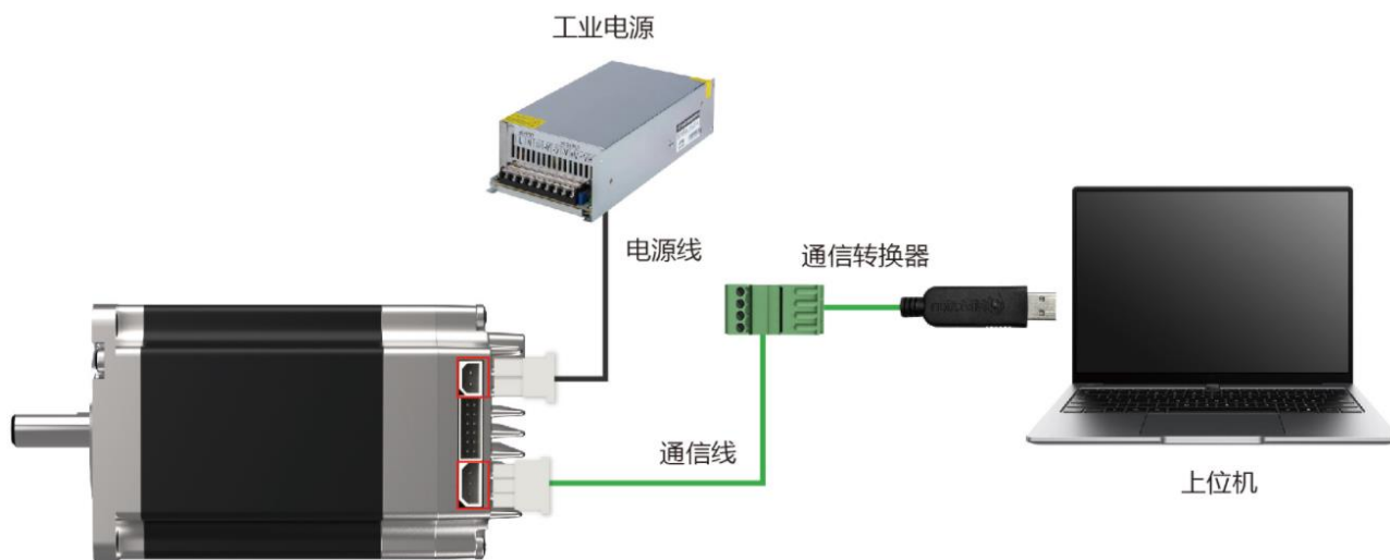
图 16 一体化电机调试接线图
