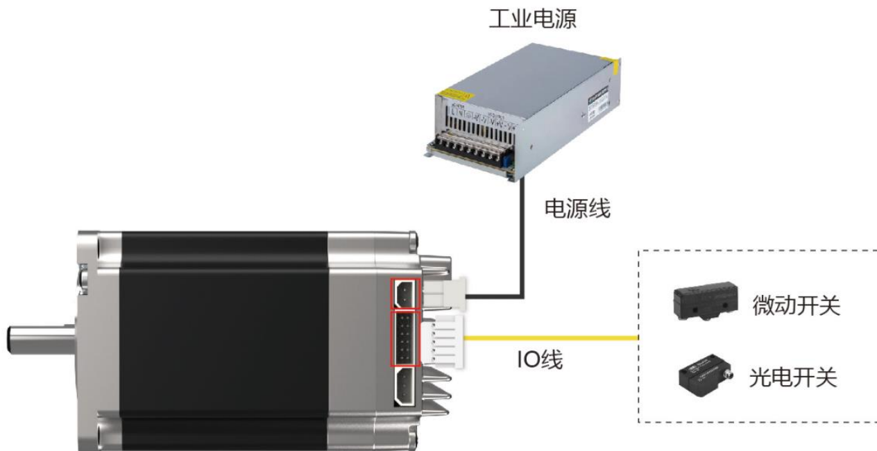
图 18 外部控制接线图（通过 IO 端口控制）
