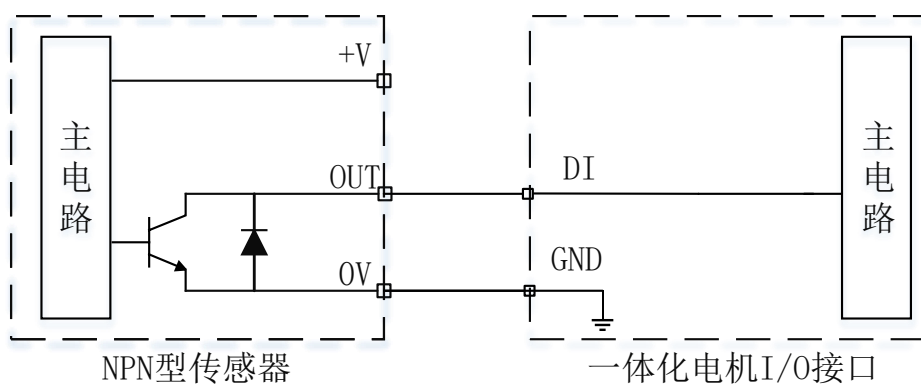
图 12 DI 输入端口接传感器示意图
