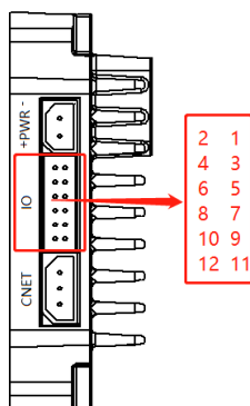
图 10 I/O 输入输出端口
