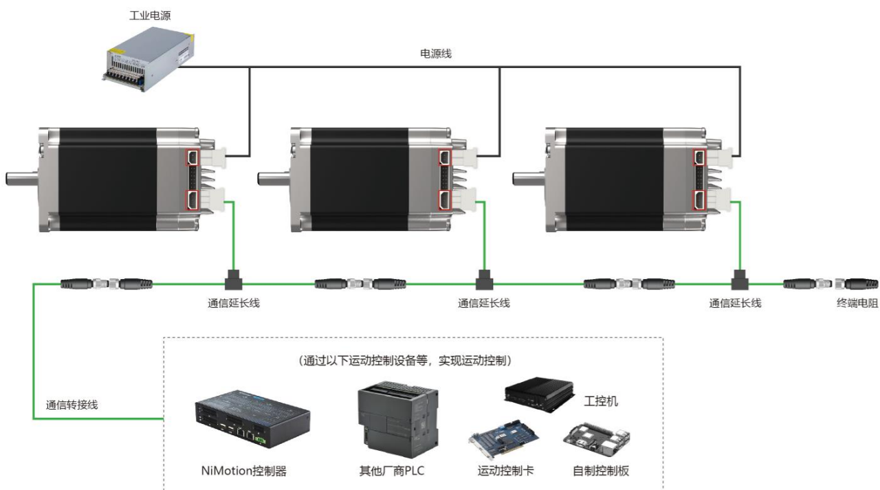
图 19 一体化电机网络拓扑图
