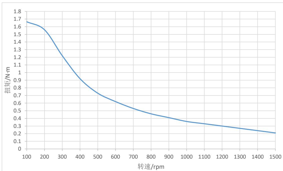
图 5 STM5776A-485-E-XX 矩频特性图（24V，2.8A，1/8 细分）
