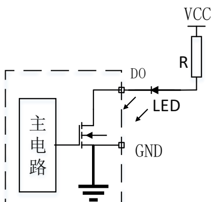
图 15 DO 输出端口接 LED 灯示意图
