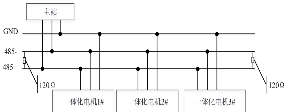
图 11 RS485 通信接线示意图
