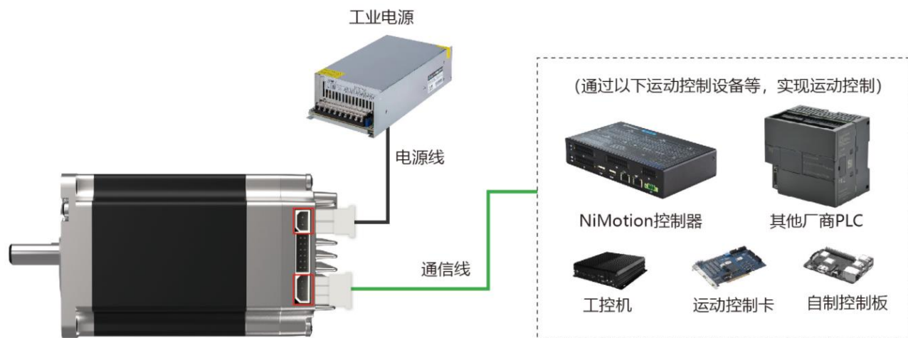
图 17 外部控制接线图（通过通信总线控制）
