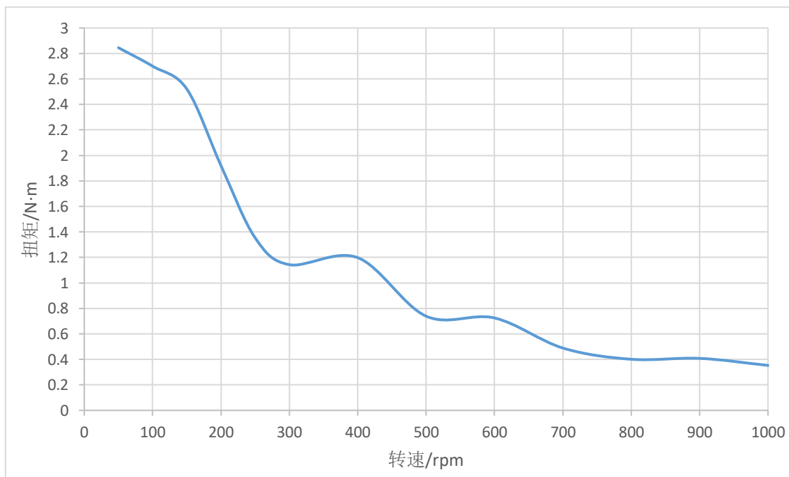
图 6 STM57B5X-CANopen-H-0FS 矩频特性图（48V，2.8A，1/8 细分）
