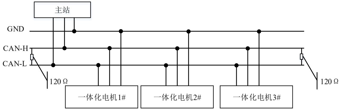
图 11 CANopen 通信接线示意图
