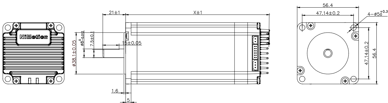
图 2 产品结构图
