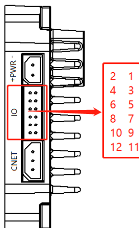
图 10 I/O 输入输出端口
