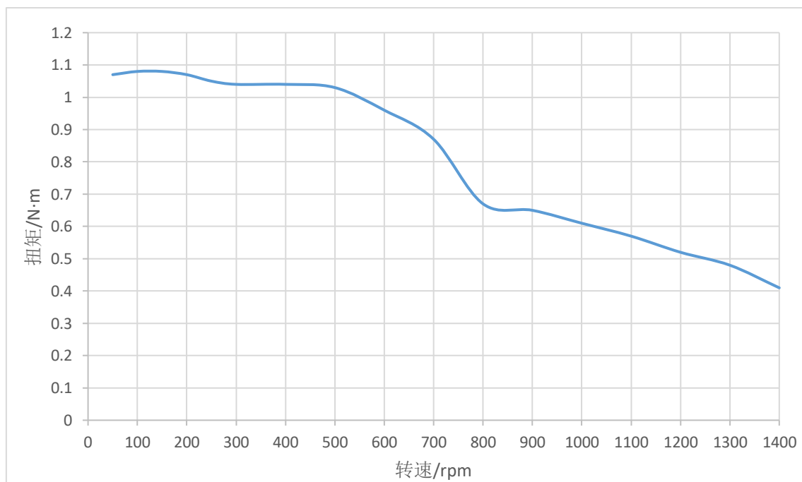
图 4 STM5756X-CANopen-H-0FS 矩频特性图（48V，2.8A，1/8 细分）
