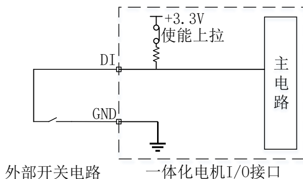
图 14 DI 输入端口接开关示意图
