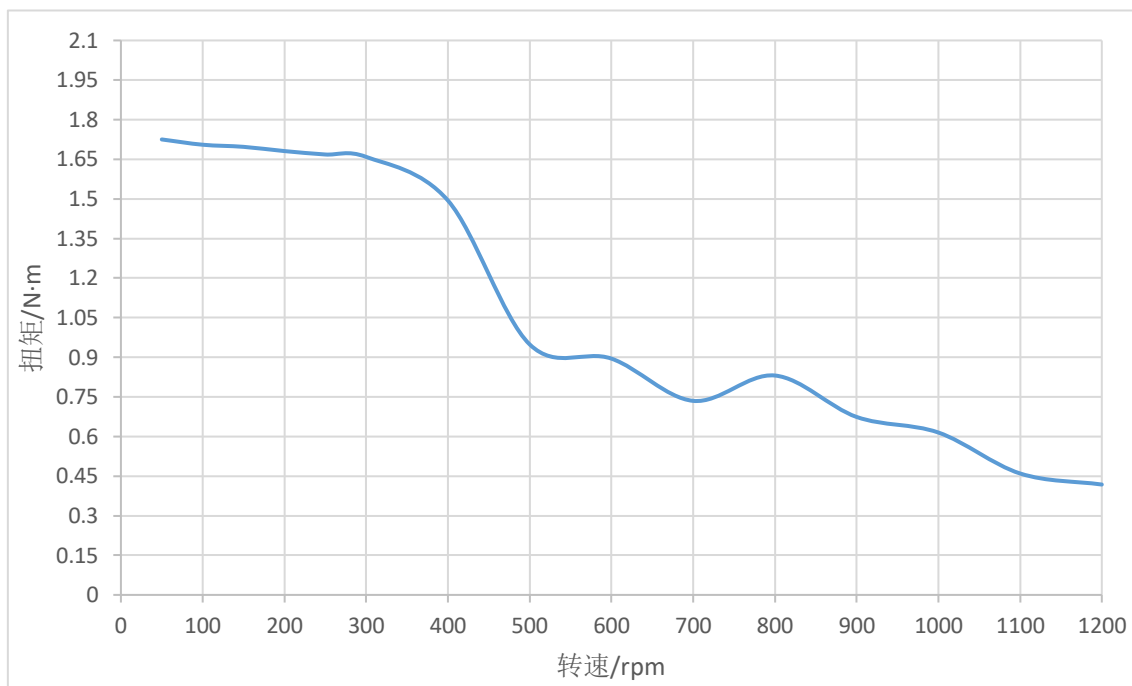
图 5 STM5776X-CANopen-H-0FS 矩频特性图（48V，2.8A，1/8 细分）
