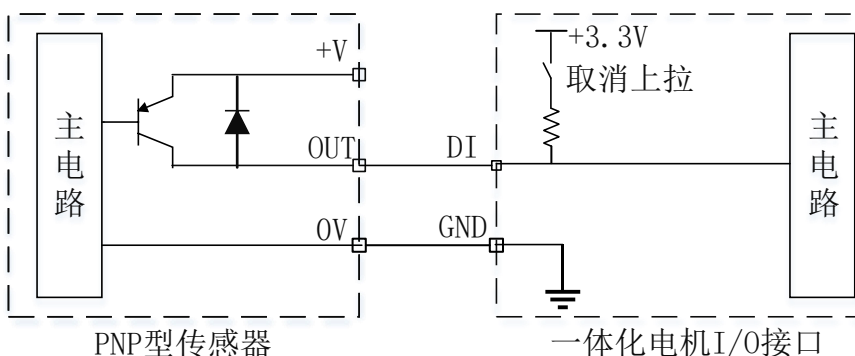
图 13 DI 输入端接 PNP 型传感器示意图
