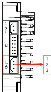
图 9 通信端口
