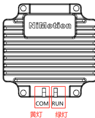
图 7 指示灯
