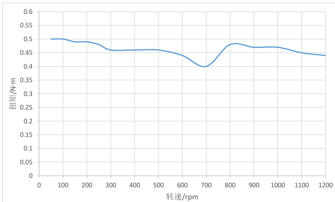
图 3 STM5741X-CANopen-H-0FS 矩频特性图（48V，2.8A，1/8 细分）
