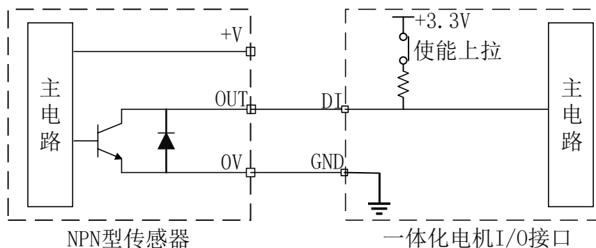
图 12 DI 输入端口接 NPN 型传感器示意图
