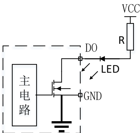
图 15 DO 输出端口接 LED 指示灯示意图
