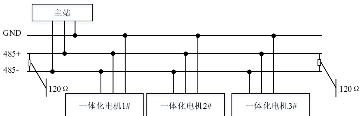
图 4-1 RS485 通信接线拓扑图
