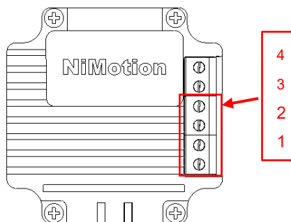
图 3-3 相线接口
