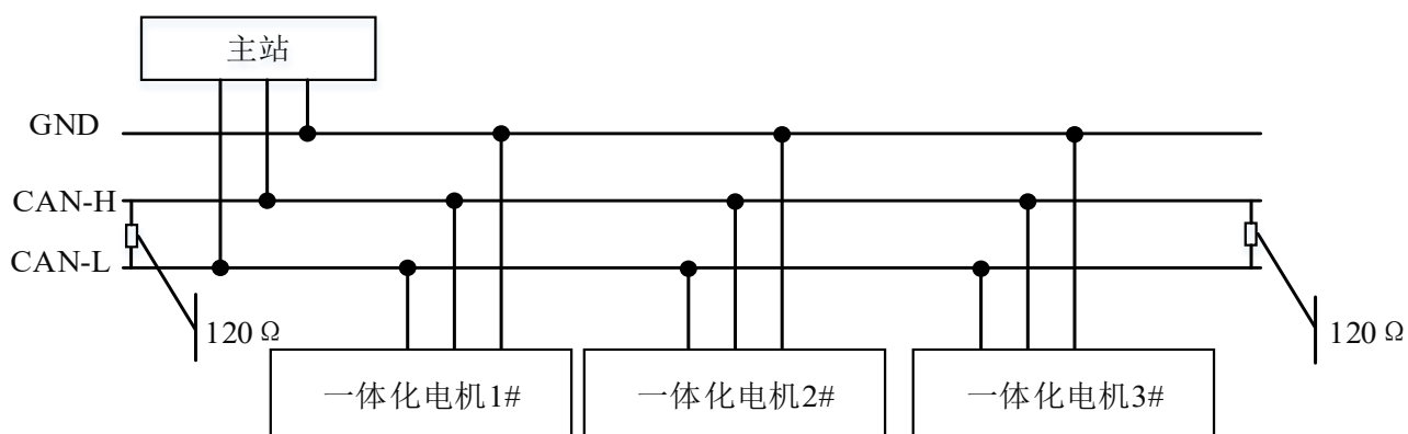
图 4-2 CANopen 通信接线示意图
