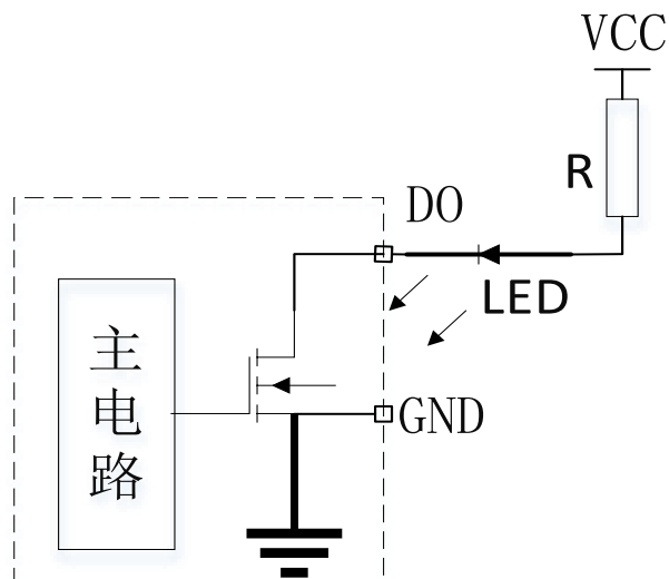
图 3-9 DO 输出端口接 LED 指示灯示意图
