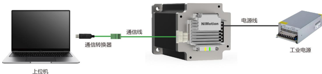
图 4-2 一体化电机调试接线图
