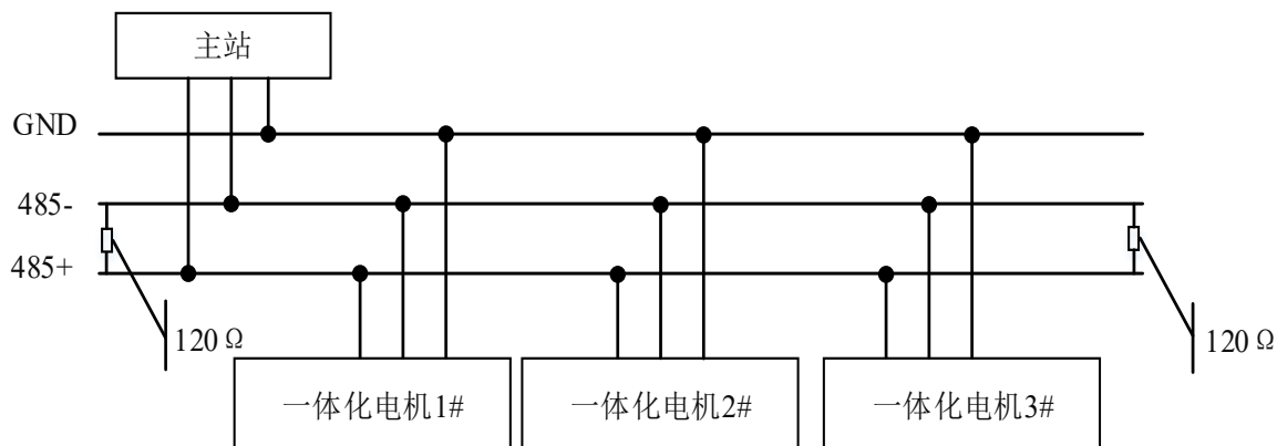
图 4-2 RS485 通信接线示意图
