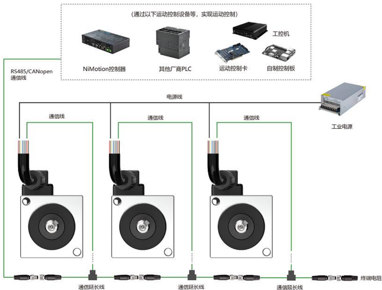
图 4-5 组网拓扑图
