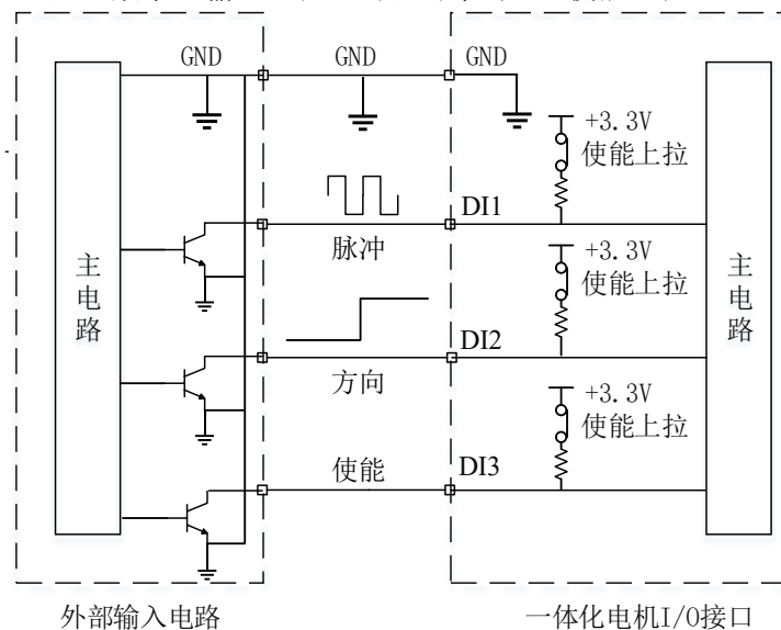
图 3-4 DI 接脉冲输入示意图
