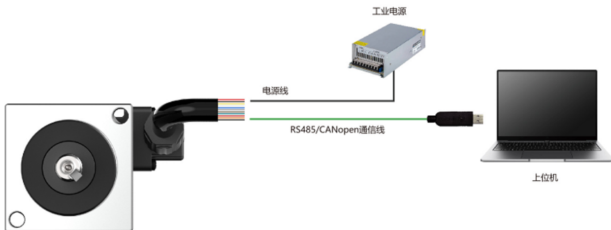
图 4-3 一体化电机调试接线图
