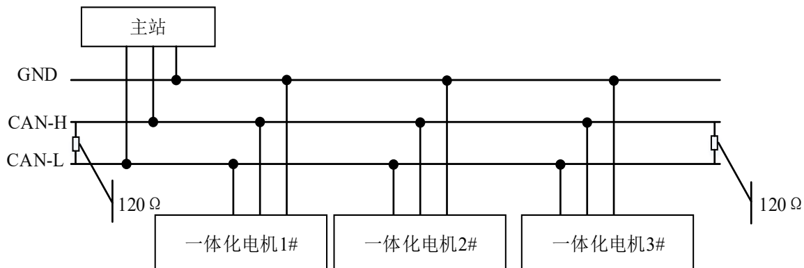
图 4-1 CANopen 通信接线示意图
