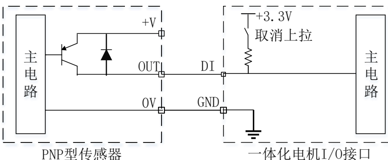
图 3-2 DI 输入端口接 PNP 型传感器示意图
