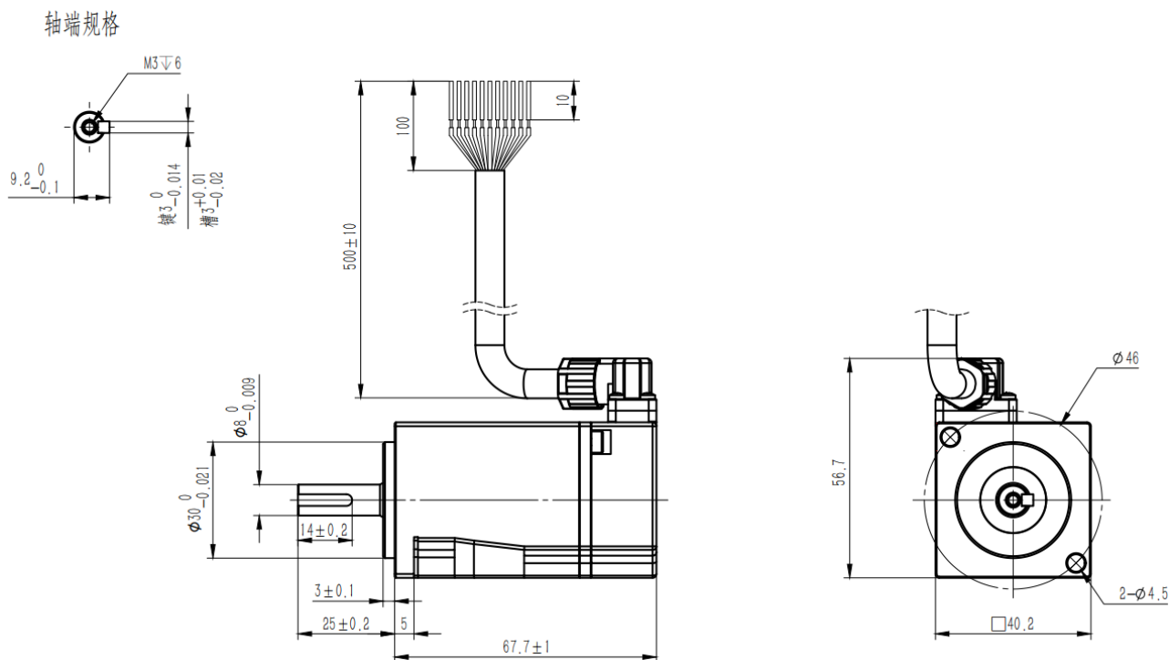
图 2-2 产品结构图
