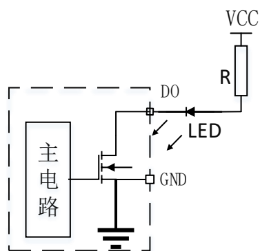
图 3-5 DO1 输出端口接 LED 指示灯示意图
