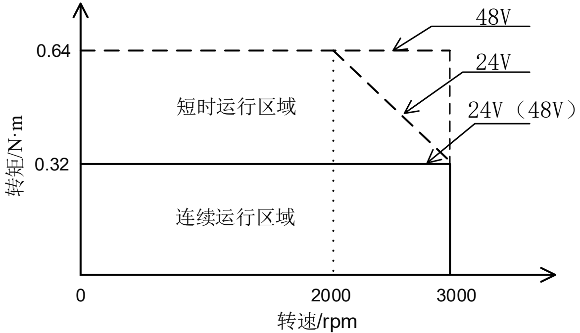
图 2-3 PMMP4010B-CANopen/485-L-XX 矩频特性图 (6.5A)
