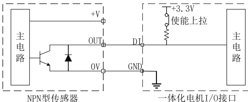
图 3-1 DI 输入端口接 NPN 型传感器示意图
