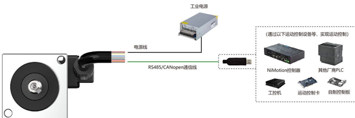
图 4-4 外部控制接线图
