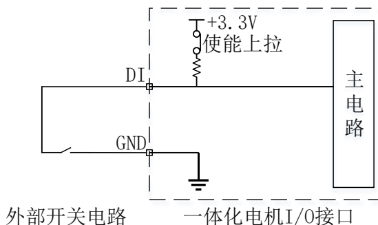
图 3-3 DI 输入端口接开关示意图
