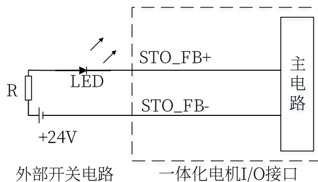
图 3-13 STO 反馈接线示意图（接 LED）
