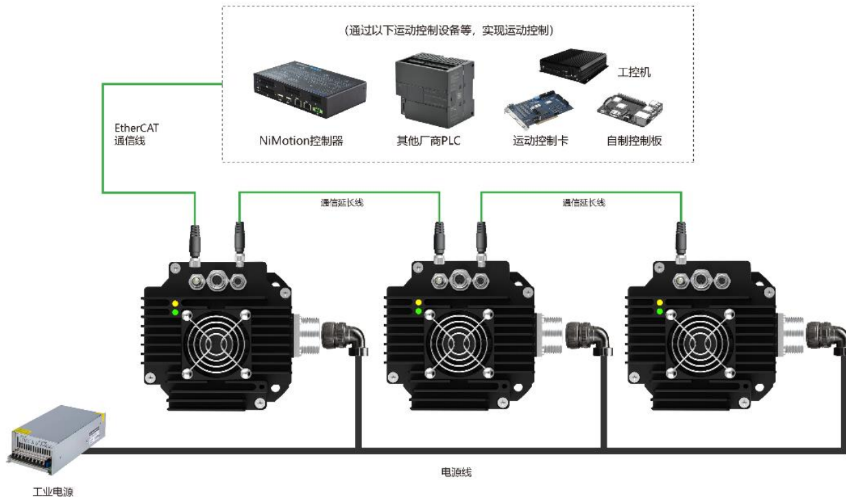
图 4-9 EtherCAT 通信组网接线图
