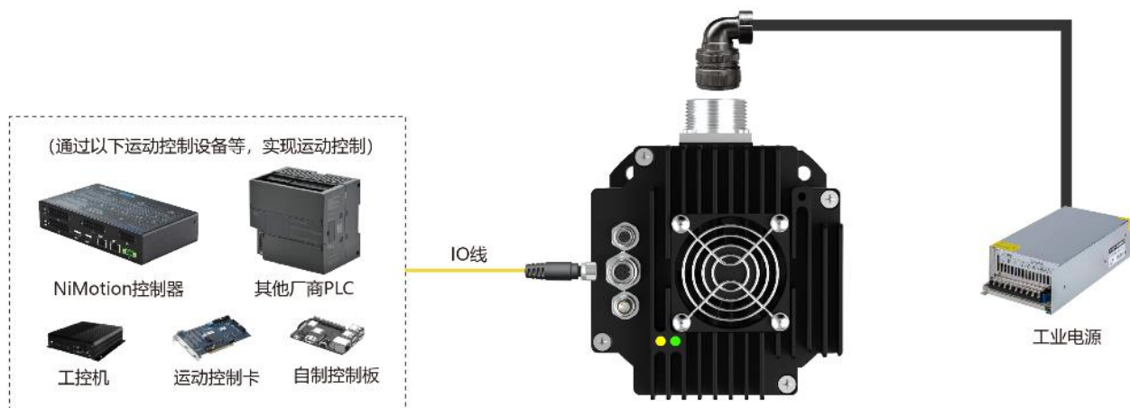
图 4-6 外部控制接线图
