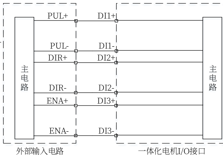
DI1、DI2、DI3（输入端）接脉冲输入
