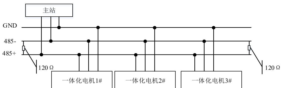
图 4-3 RS485 通信接线拓扑图
