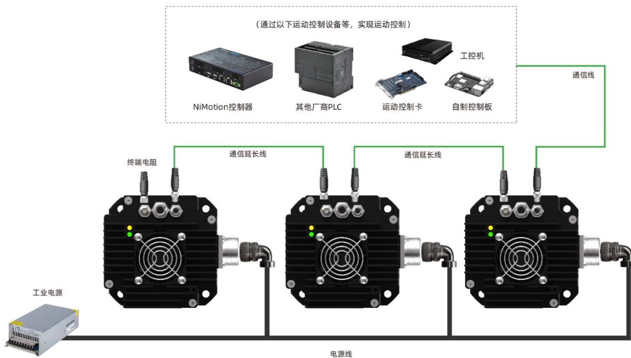
图 4-8 RS485&CANopen 通信组网接线图
