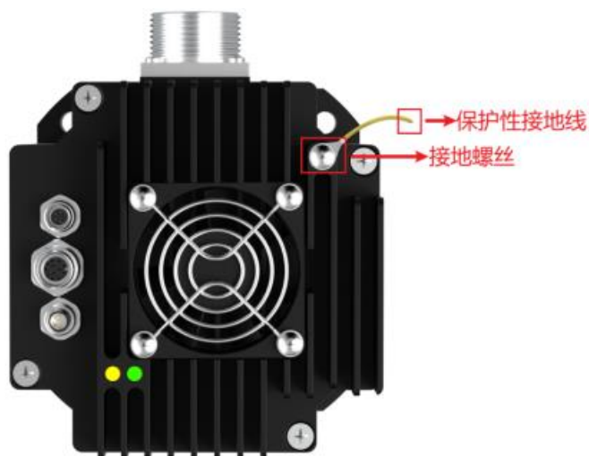
图 3-4 外壳保护性接地示意图
