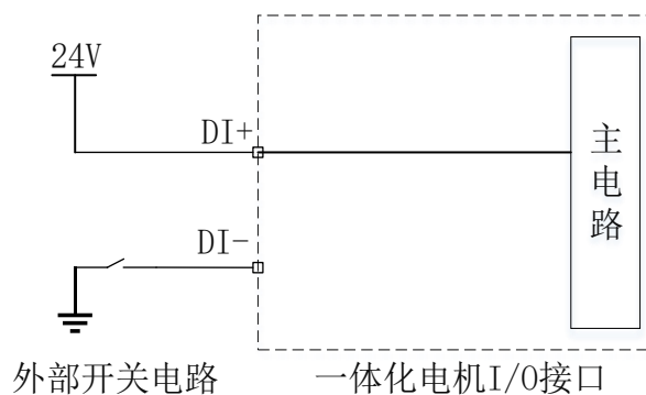
图 3-9 DI 输入端口接开关示意图
