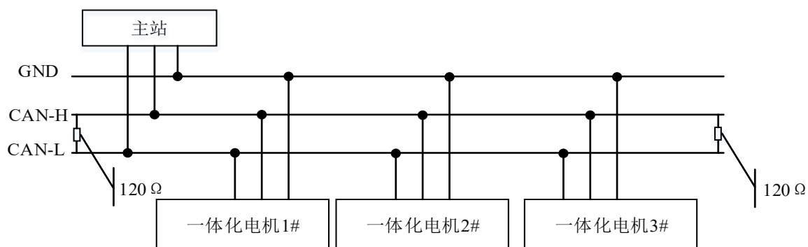
图 4-2 CANopen 通信接线拓扑图
