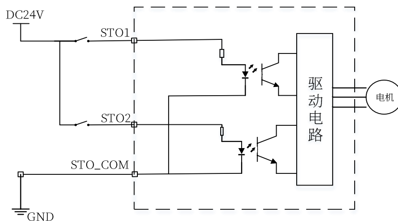
图 3-14 STO 功能接线示意图
