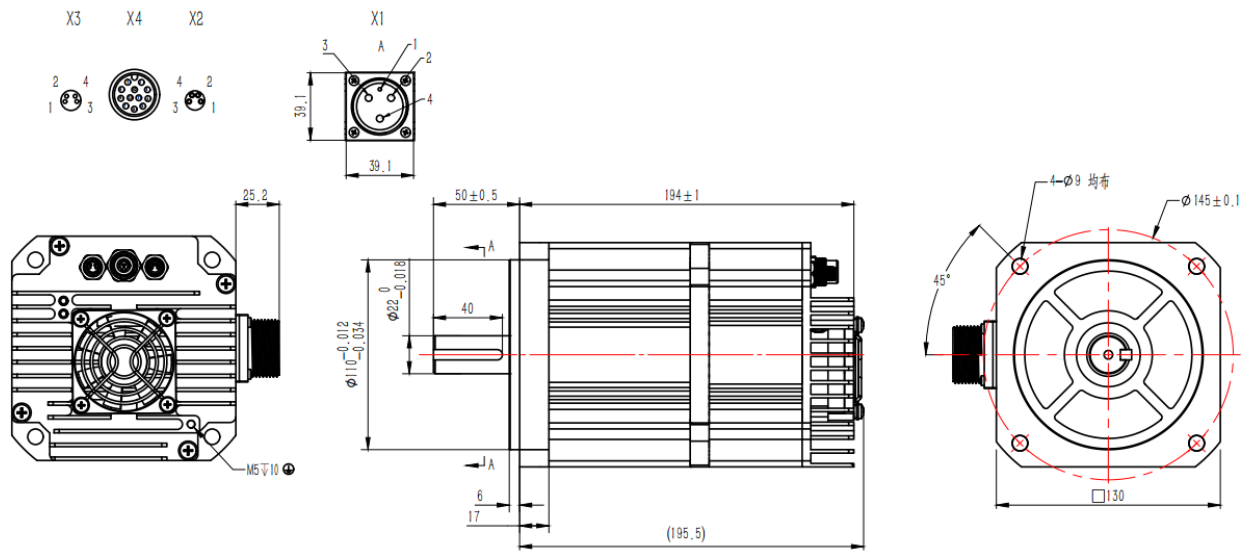
图 2-2 PSMP130 系列（标准款）产品结构图
