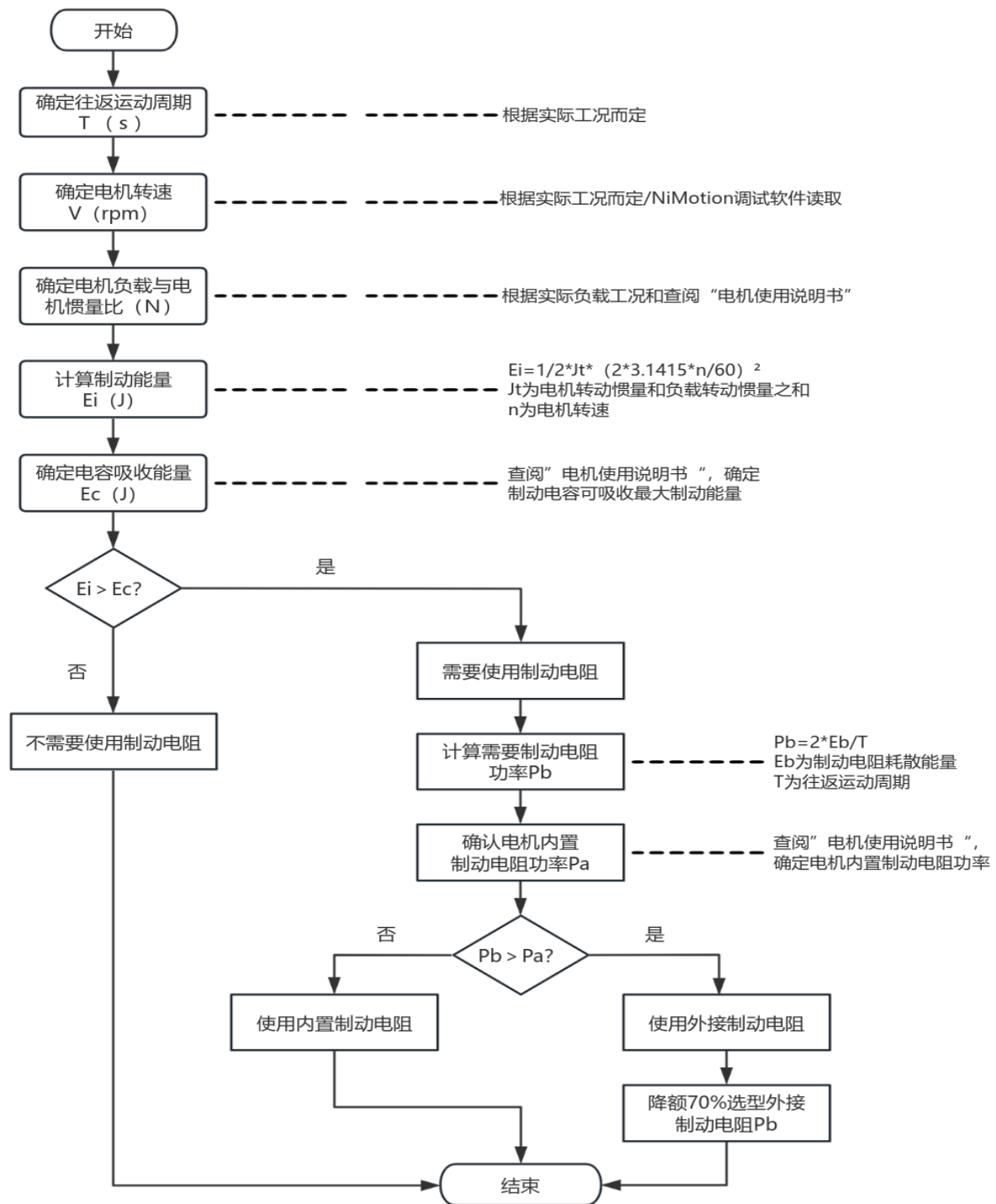
图 5-1 制动电阻选型流程图
