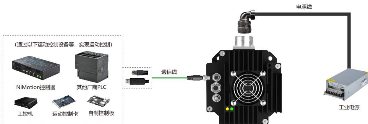
图 4-5 外部控制接线图
