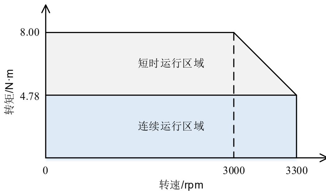
图 2-4 PSMP1301K5X-COE/CANopen/485-XX 矩频特性图（48V，45A）
