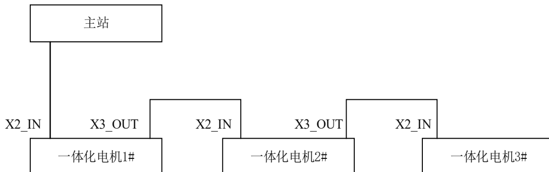
图 4-1 EtherCAT 通信接线拓扑图
