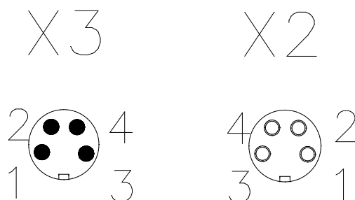
图 3-5 通信端口
