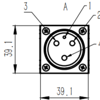
图 3-2 电源端口
