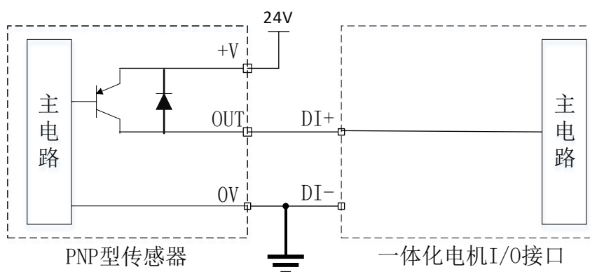
图 3-8 DI 输入端口接 PNP 型传感器示意图
