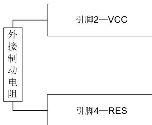
图 3-3 外接制动电阻接线图
