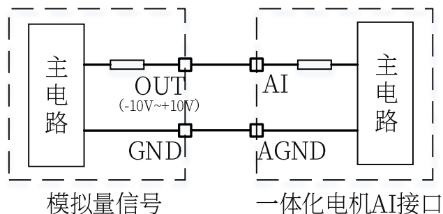
图 3-12 AI 端口接模拟量输入示意图
