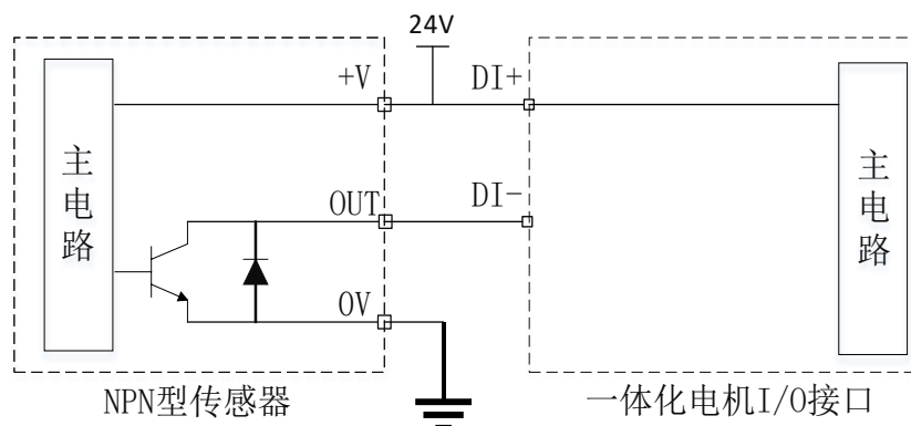
图 3-7 DI 输入端口接 NPN 型传感器示意图
