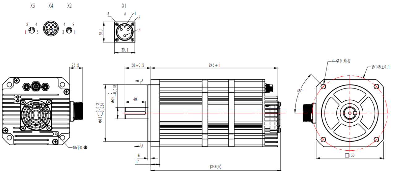
图 2-3 PSMP130 系列（带制动器款）产品结构图
