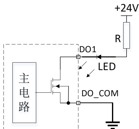
图 3-11 DO1 输出端口接 LED 指示灯示意图
