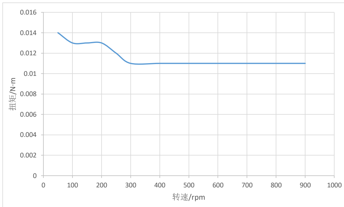
图 2-3 STM2033X-CANopen/485-M-XX 矩频特性图 (24V, 1.0A)
