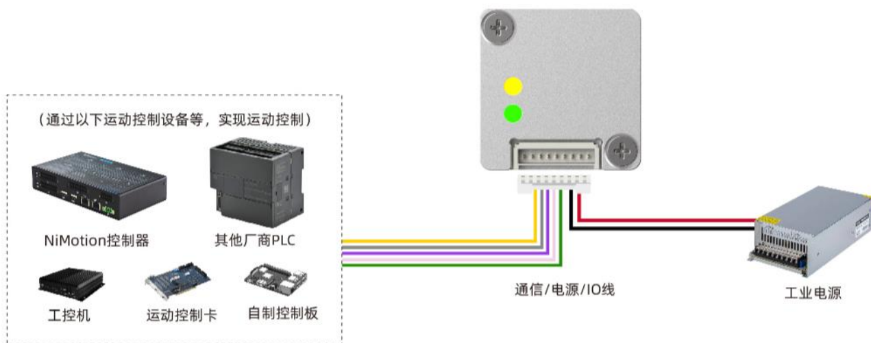
图 4-5 外部控制接线图
