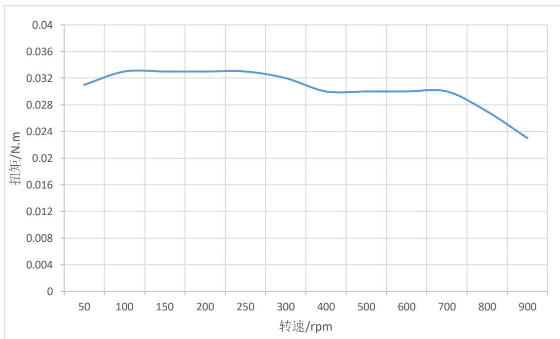
图 2-4 STM2038X-CANopen/485-M-XX 矩频特性图 (24V, 1.0A)
