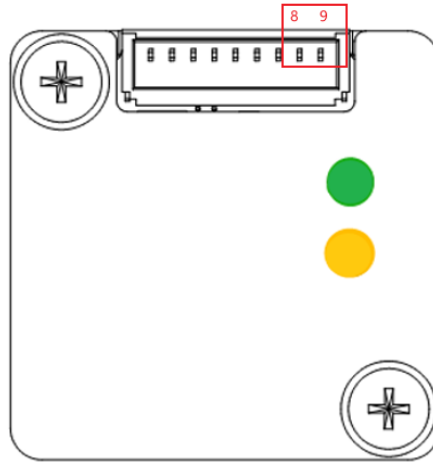
图 3-3 通信端口
