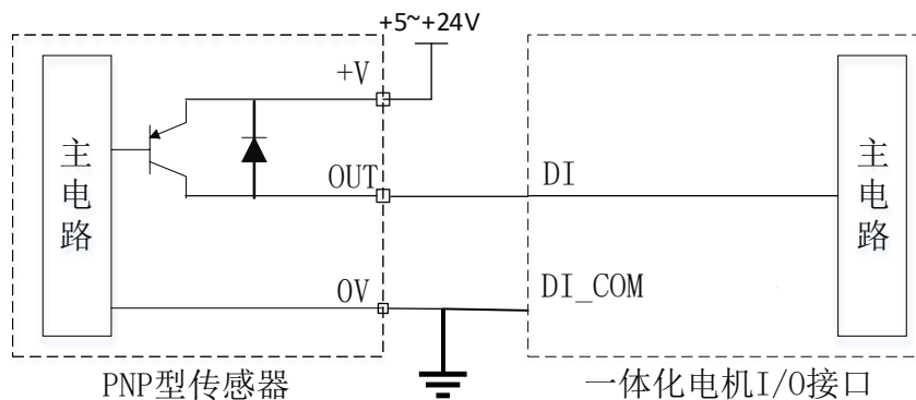
图 3-5 DI 输入端口接 PNP 型传感器示意图
