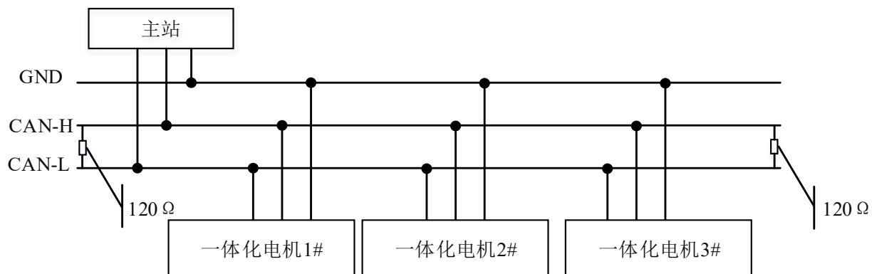
图 4-1 CANopen 通信接线拓扑图
