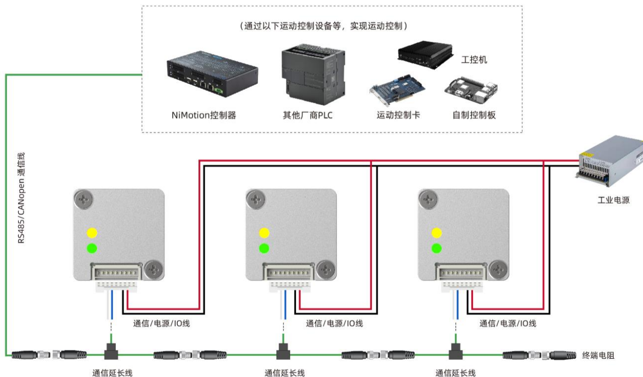
图 4-7 RS485&CANopen 通信组网接线图
