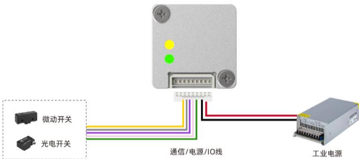
图 4-6 外部控制接线图
