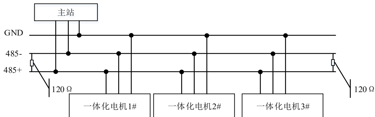
图 4-2 RS485 通信接线拓扑图
