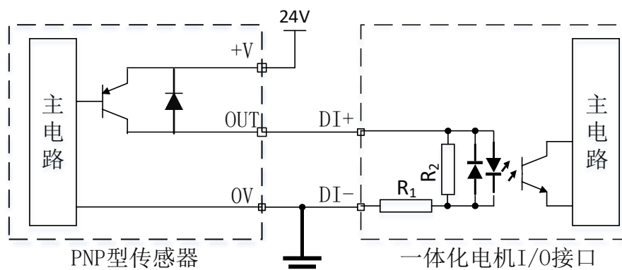
图 3-6 DI 输入端口接 PNP 型传感器示意图
