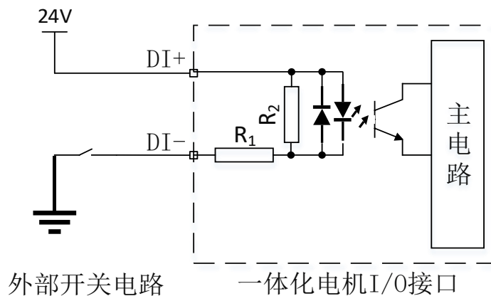
图 3-7 DI 输入端口接开关示意图
