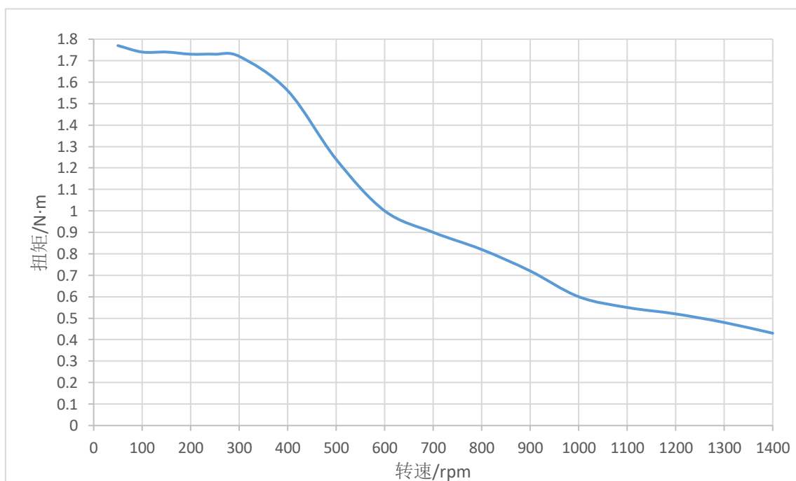
图 2-4 STMPW5776X-XX 矩频特性图（48V，4.2A）
