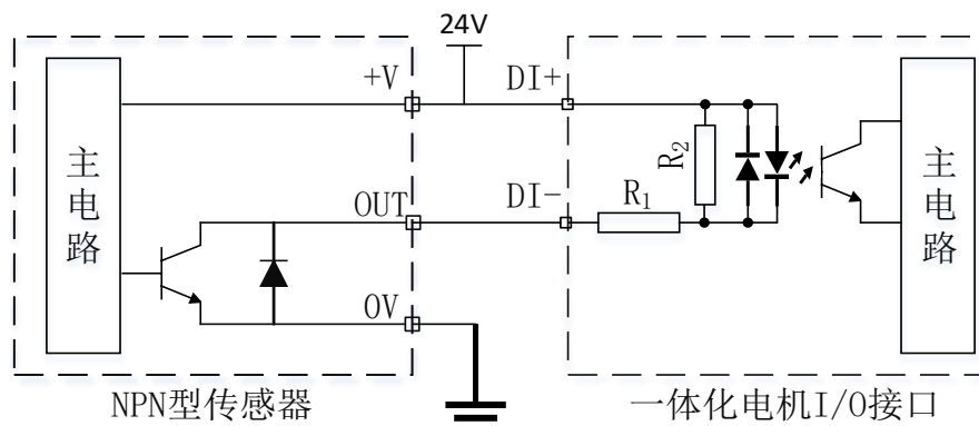
图 3-5 DI 输入端口接 NPN 型传感器示意图
