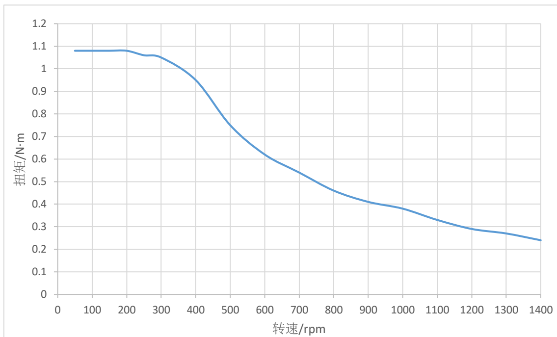
图 2-3 STMPW5756X-XX 矩频特性图（48V，3.0A）
