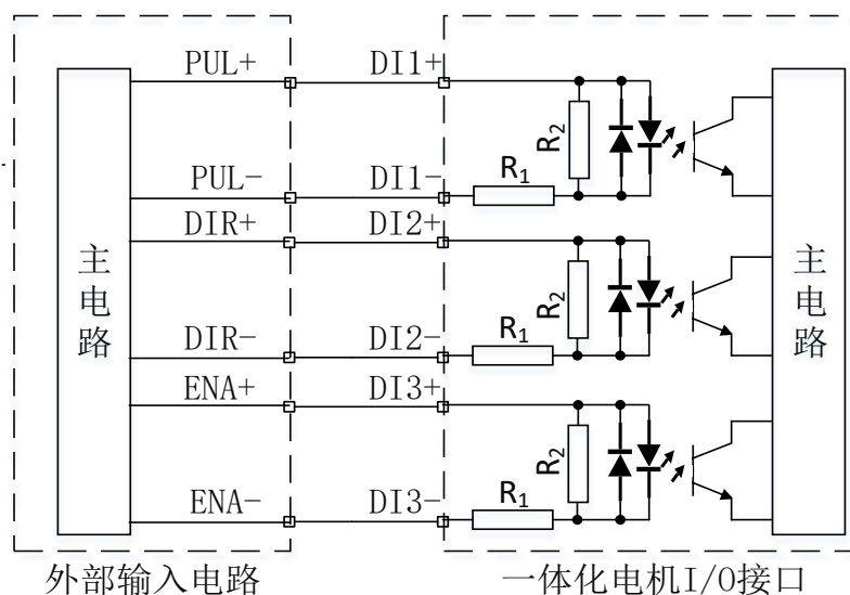
图 3-8 DI 输入端口接脉冲输入示意图
