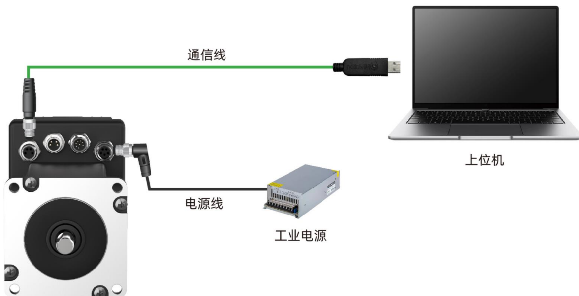
图 4-3 一体化电机调试接线图
