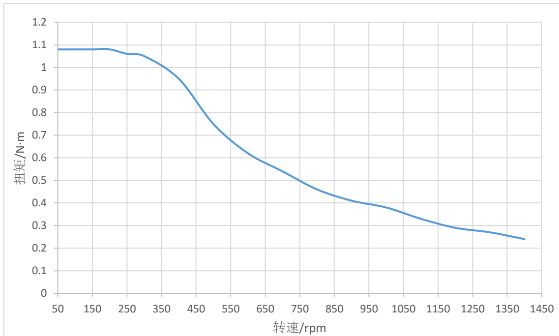
图 2-3 STMP5756X-XX 矩频特性图（48V，3.0A）
