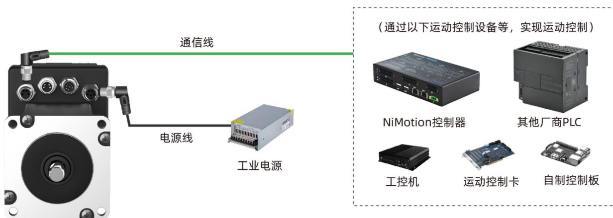
图 4-4 外部控制接线图（通过通信总线控制）
