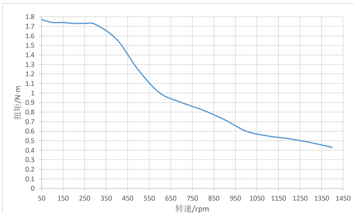
图 2-4 STMP5776X-XX 矩频特性图（48V，4.2A）
