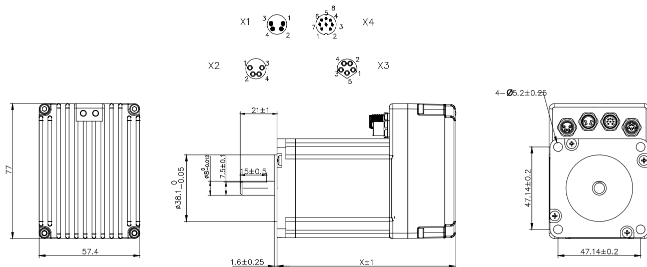
图 2-2 产品结构图
