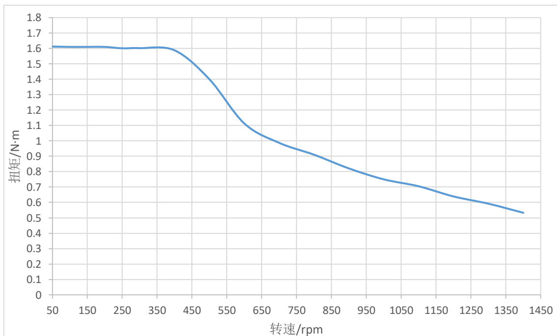
图 2-4 STMP5776X-XX 矩频特性图（48V，5.0A）
