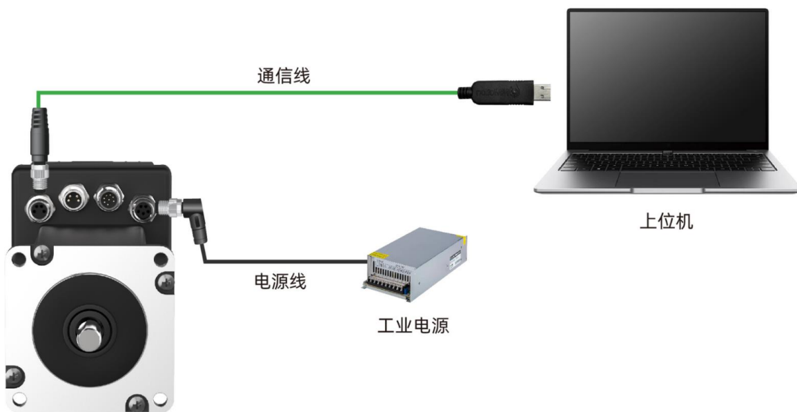
图 4-3 一体化电机调试接线图
