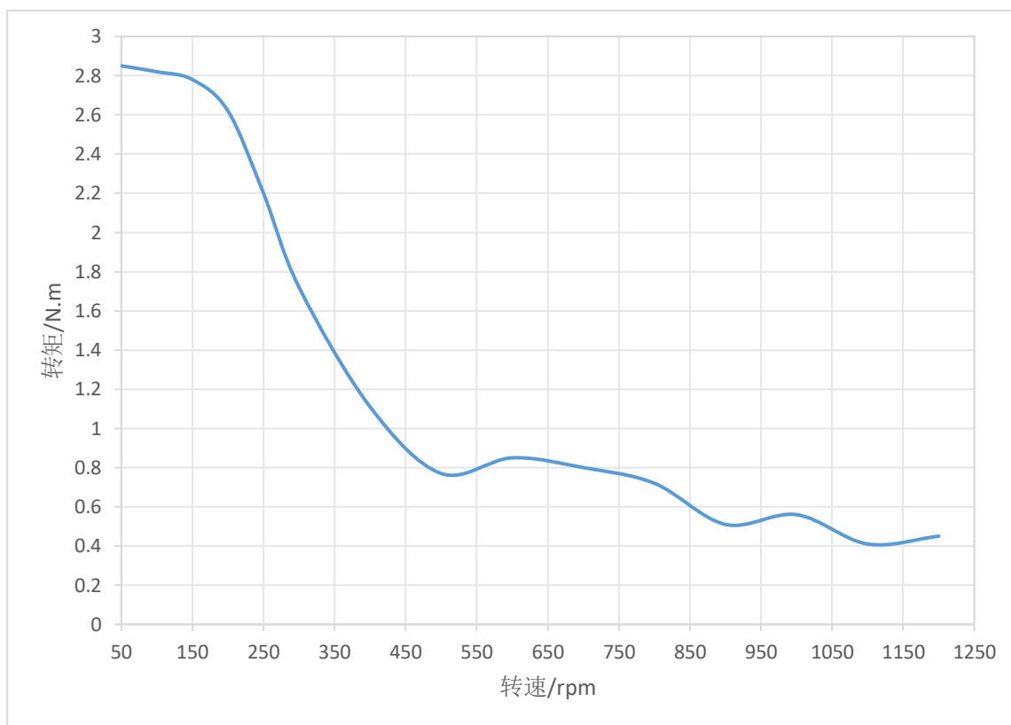
图 2-5 STMP57B5X-XX 矩频特性图 (48V, 6.0A)
