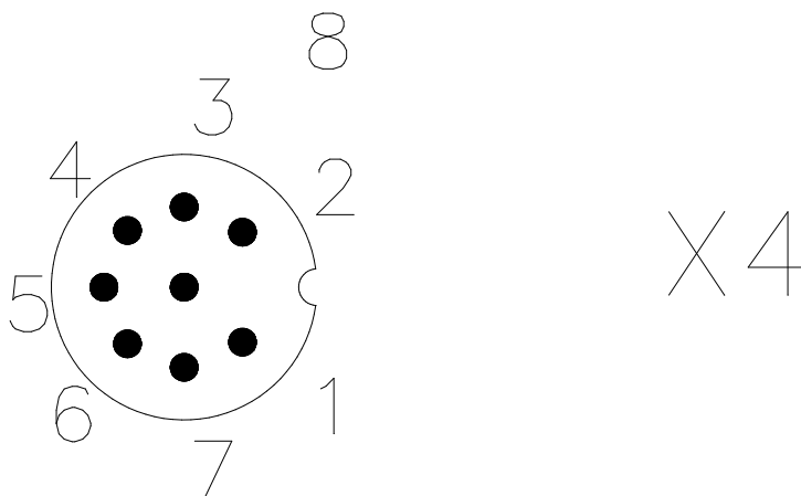
图 3-4 I/O 输入输出端口
