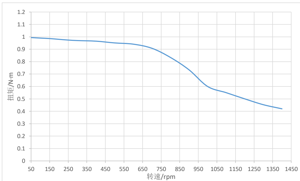
图 2-3 STMP5756X-XX 矩频特性图（48V，5.0A）
