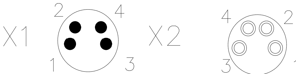
图 3-3 通信端口
