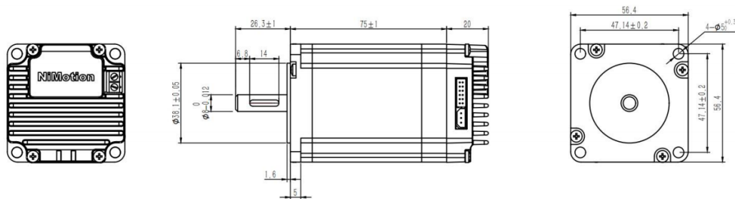
STM57ME-1FH 系列产品结构图
