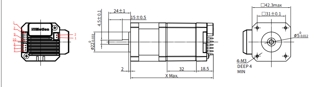
STM42 系列产品结构图 (制动器款)
