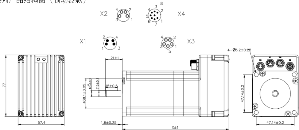
STMP57M 系列产品结构图 (制动器款)
