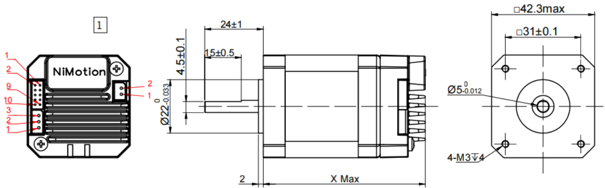
STM42M 系列产品结构图
