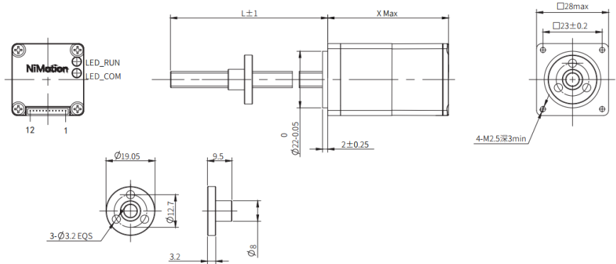
STM28-M 丝杆系列产品结构图
