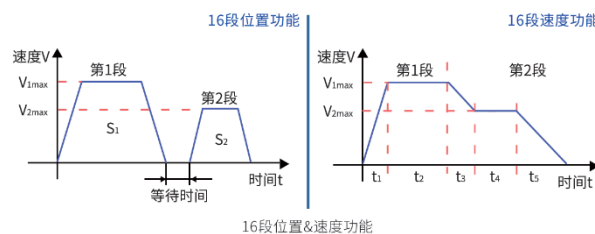
16段位置&速度功能
