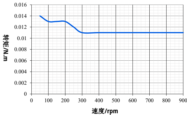
STM2033B-CANopen/485-M
