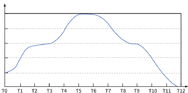
12段S型加减速曲线
