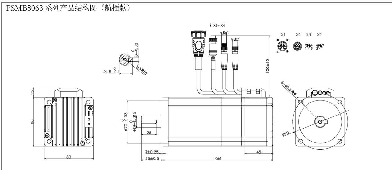
PSM(L)8075 系列产品结构图
