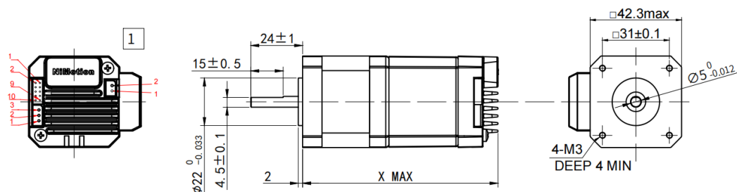
STM42M 系列产品结构图 (制动器款)
