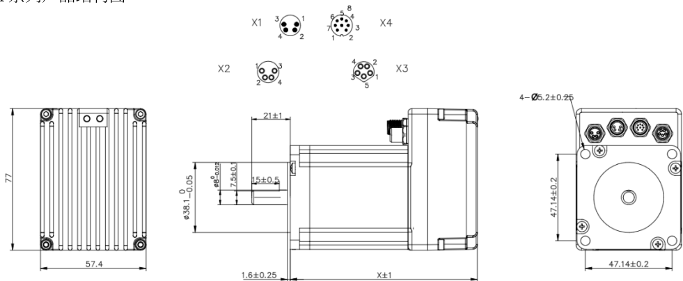
STMP57M 系列产品结构图
