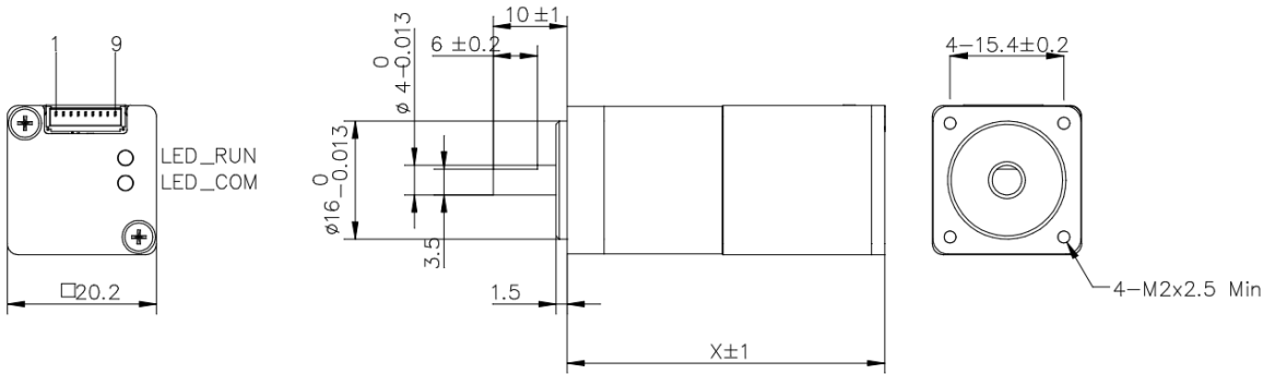
STM20M 系列产品结构图
