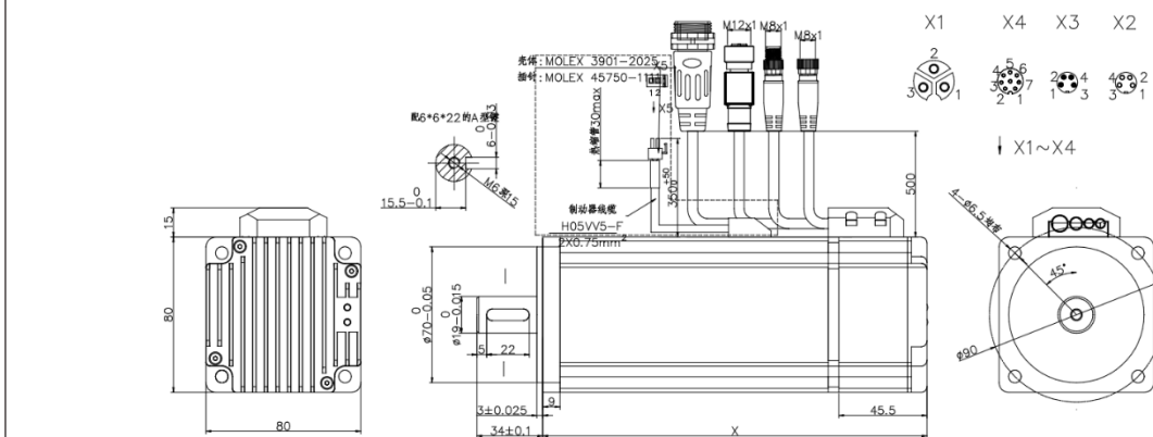
PMM8075 系列产品结构图（航插款）
