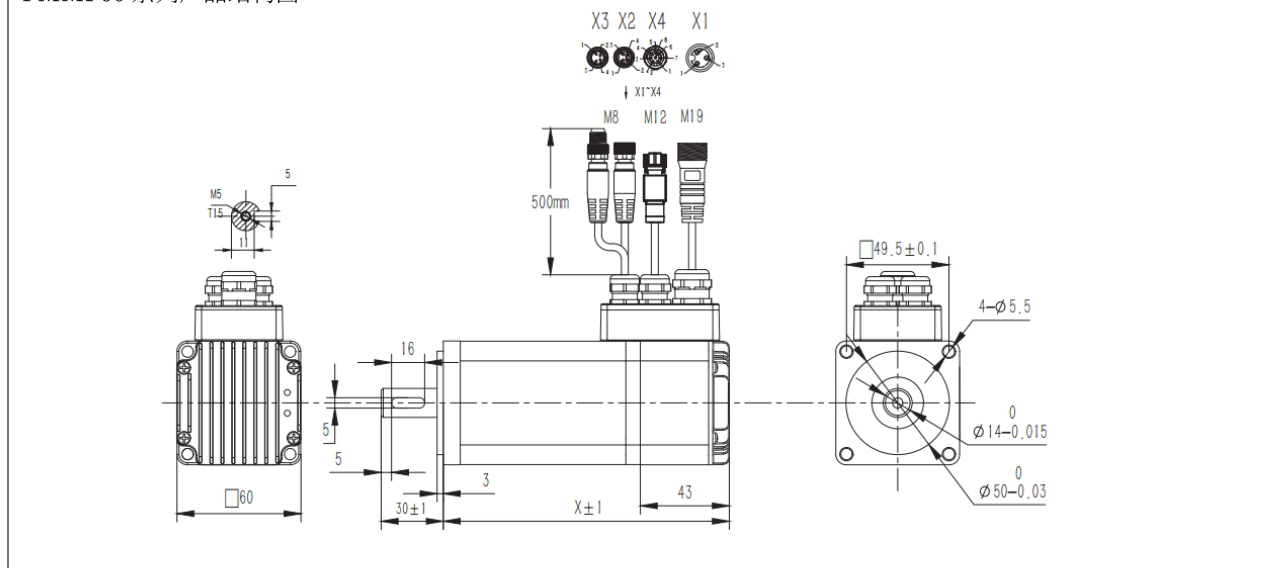
PMMP60 系列产品结构图
