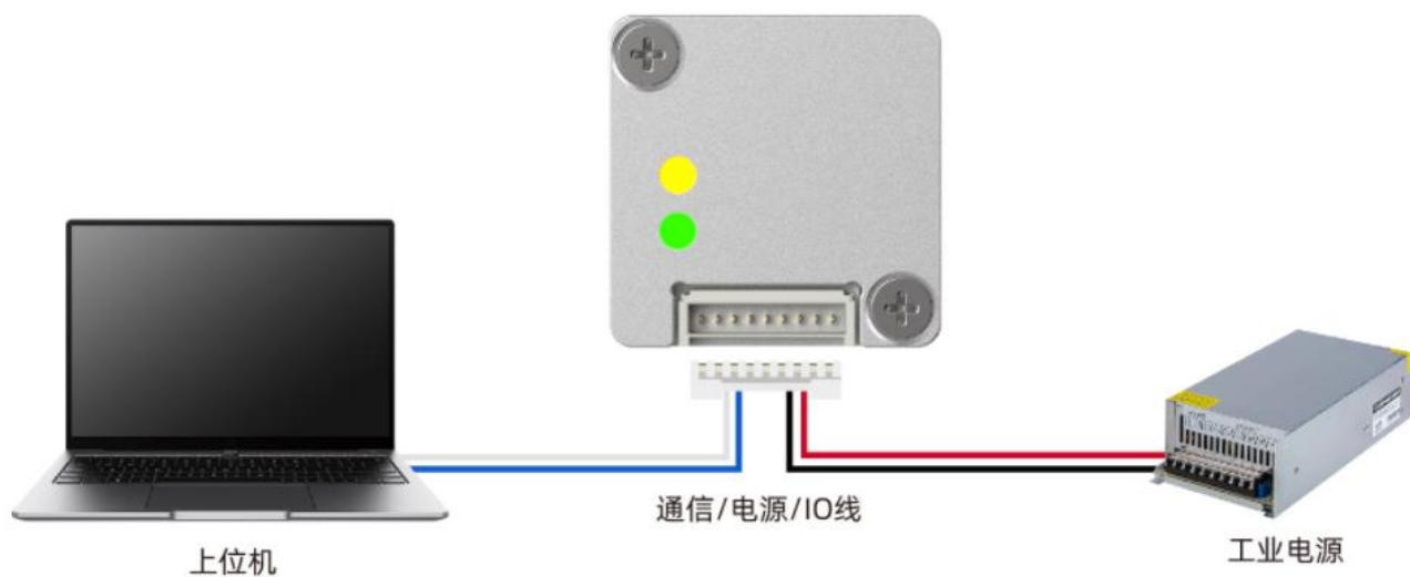
图 4-3 一体化电机调试接线图
