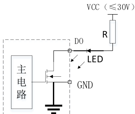
图 3-8 DO 输出端口接 LED 指示灯示意图
