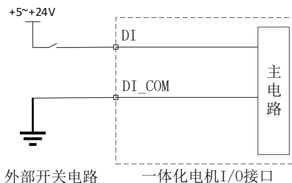
图 3-6 DI 输入端口接开关示意图
