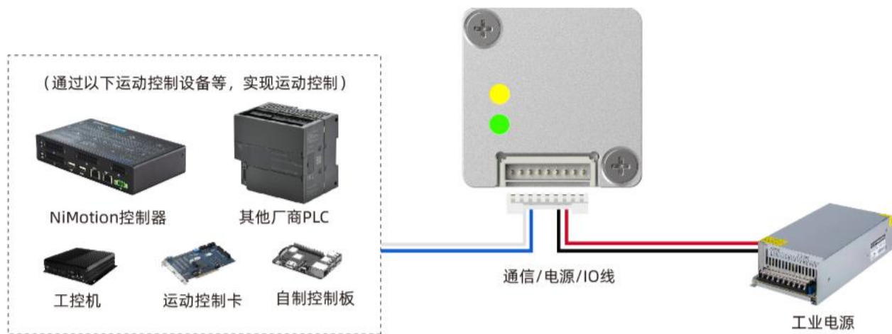
图 4-4 外部控制接线图（通过通信总线控制）
