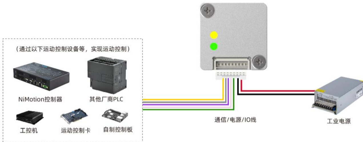
图 4-5 外部控制接线图（通过 IO 端口控制）
