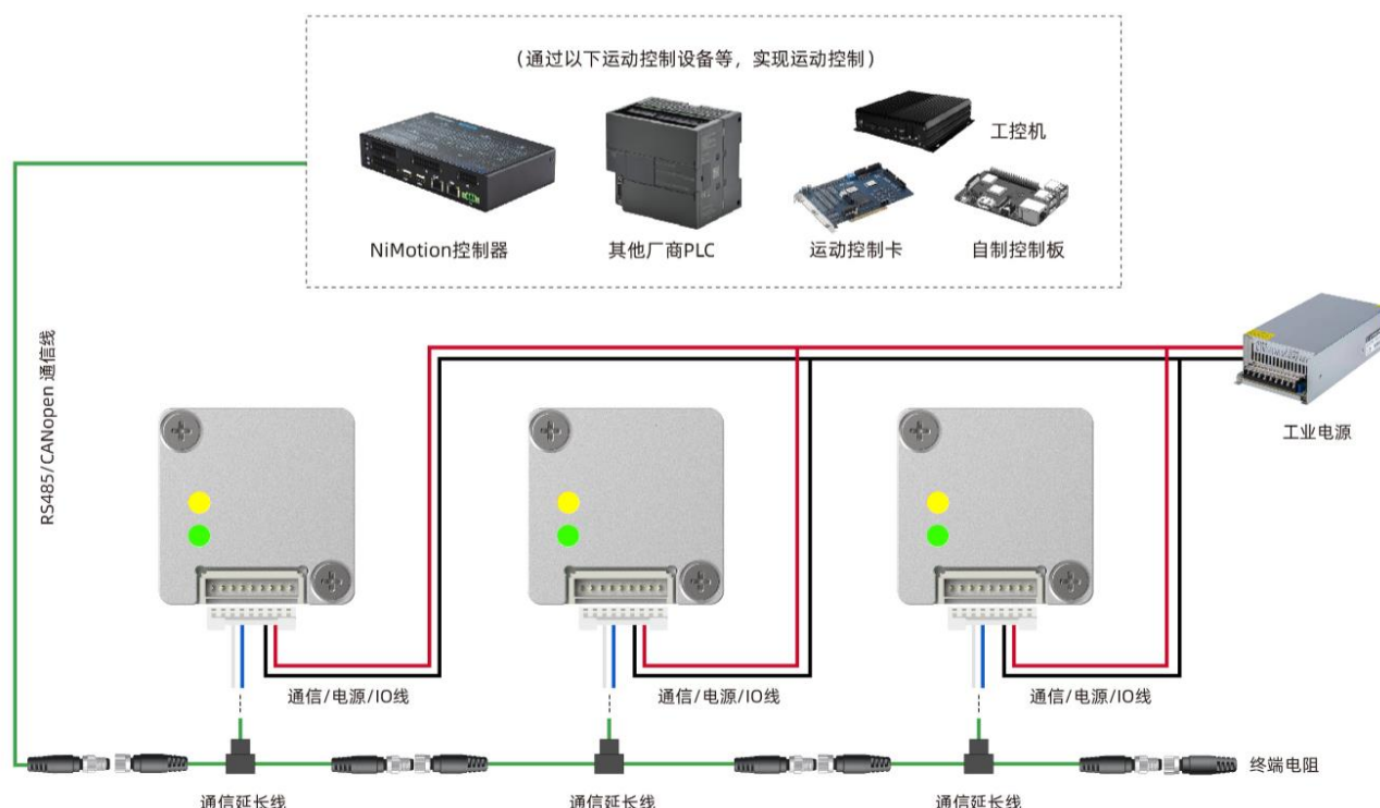
图 4-7 组网接线图 (CANopen&RS485)
