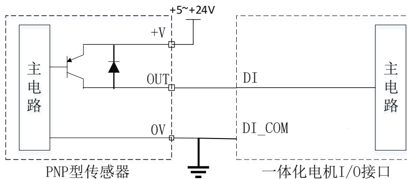
图 3-5 DI 输入端口接 PNP 型传感器示意图
