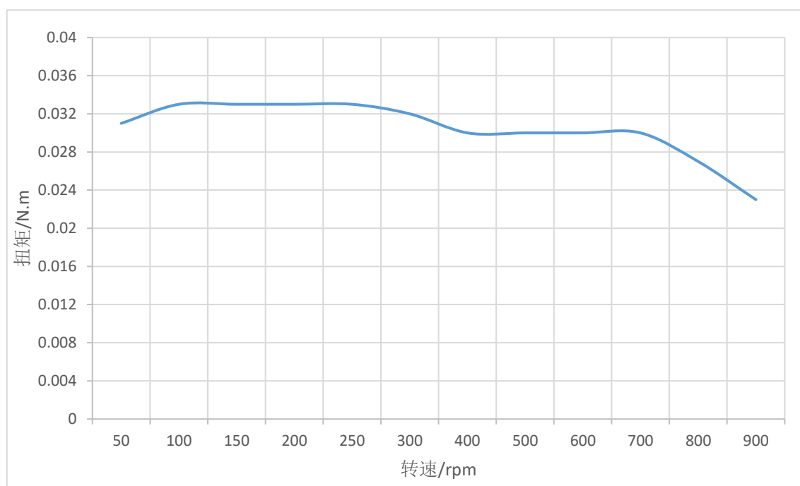
图 2-4 STM2038X-CANopen/485-M-XX 矩频特性图 (24V, 1.0A)
