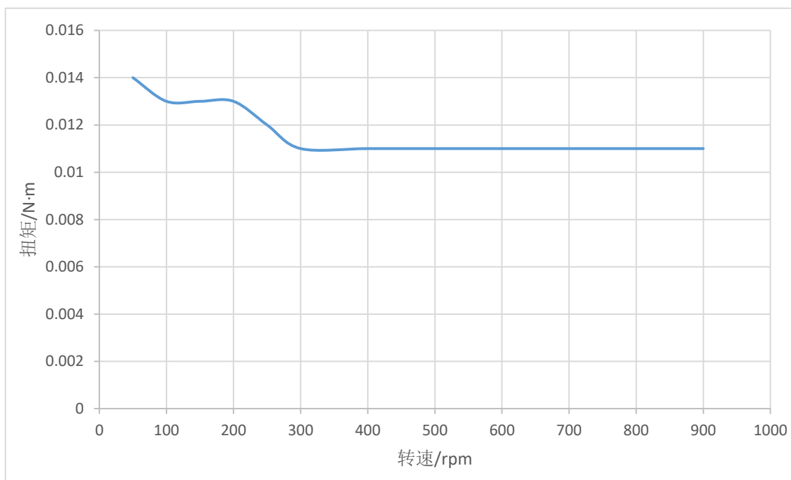
图 2-3 STM2033X-CANopen/485-M-XX 矩频特性图 (24V, 1.0A)
