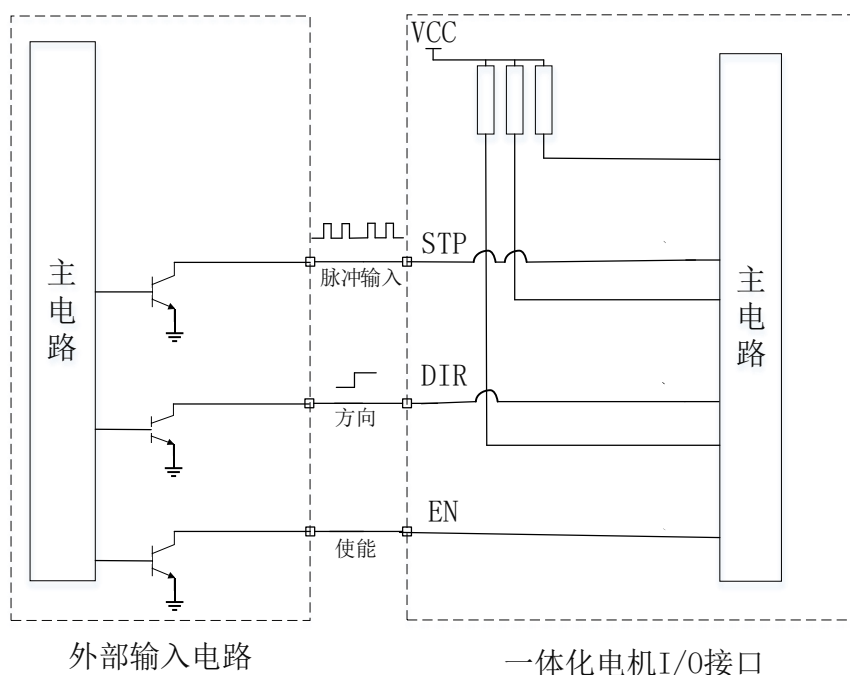
图 3-7 DI 输入端口接脉冲输入示意图
