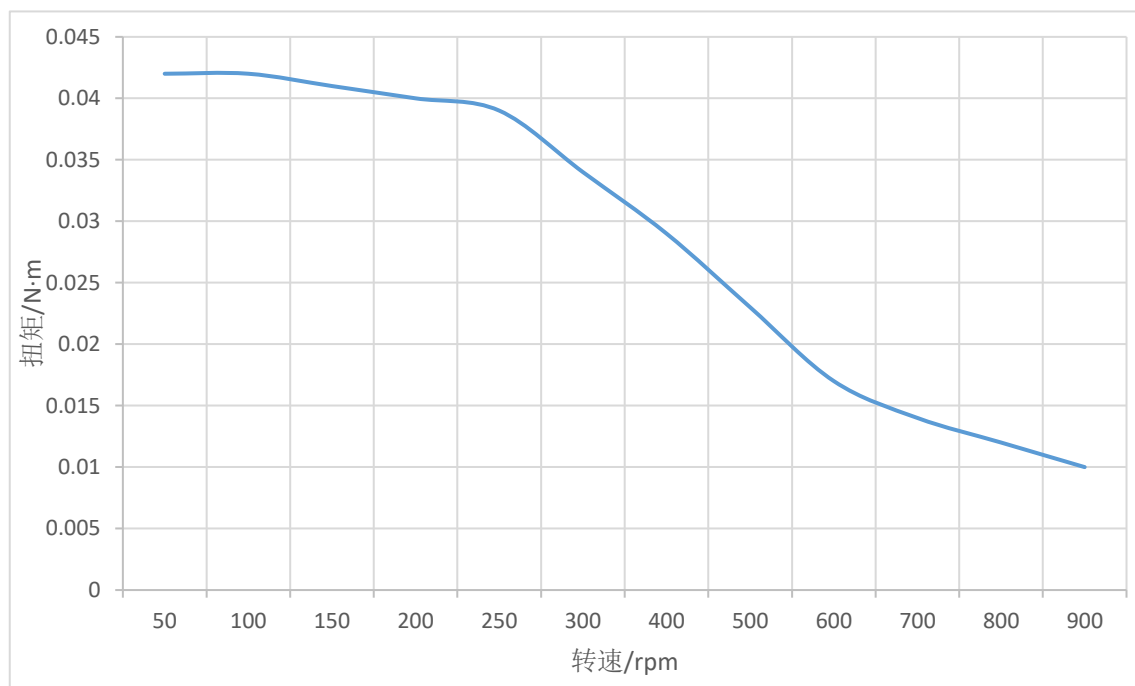
图 2-5 STM2048X-CANopen/485-M-XX 矩频特性图 (24V, 1.0A)
