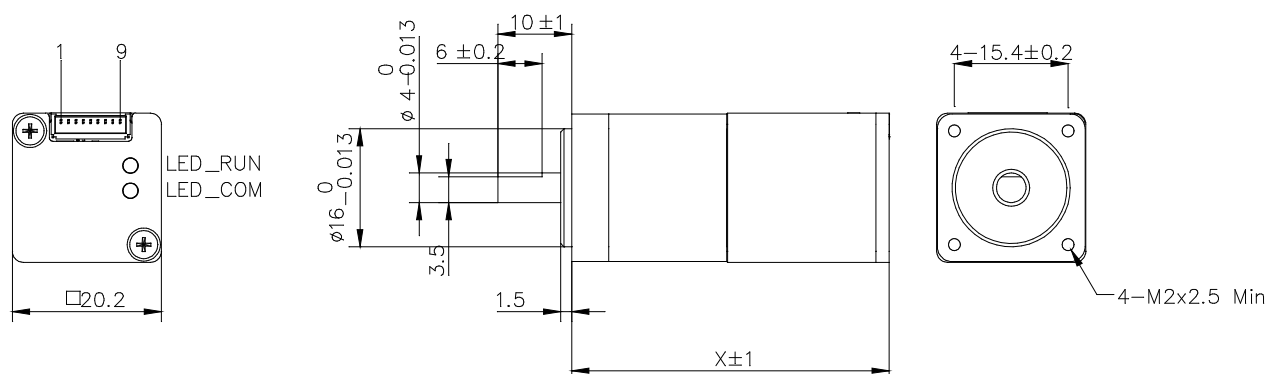
图 2-2 产品结构图
