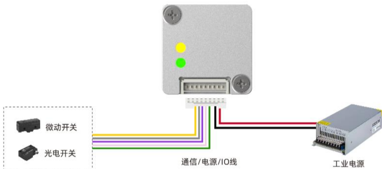
图 4-6 外部控制接线图（通过 IO 端口控制）
