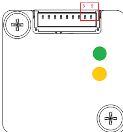
图 3-3 通信端口
